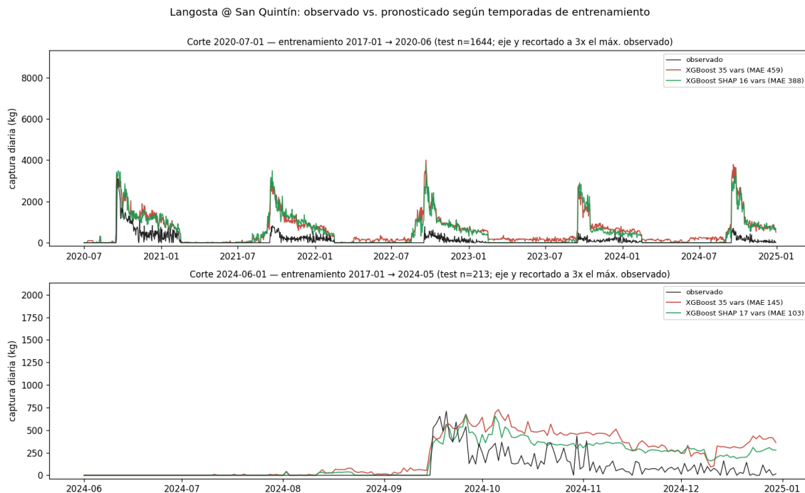
Figure 7: Langosta × San Quintín, observado (negro) vs. pronosticado por el XGBoost completo (35 vars, rojo) y el podado por SHAP (~16 vars, verde), en los dos cortes. Con el entrenamiento corto (arriba, hasta jun-2020) el modelo extrapola el régimen pre-bache y sobre-predice todas las temporadas post-2021; con el entrenamiento largo (abajo, hasta may-2024, con el bache incluido) sigue las temporadas recientes de captura reducida. Eje y recortado a 3\times el máximo observado.
