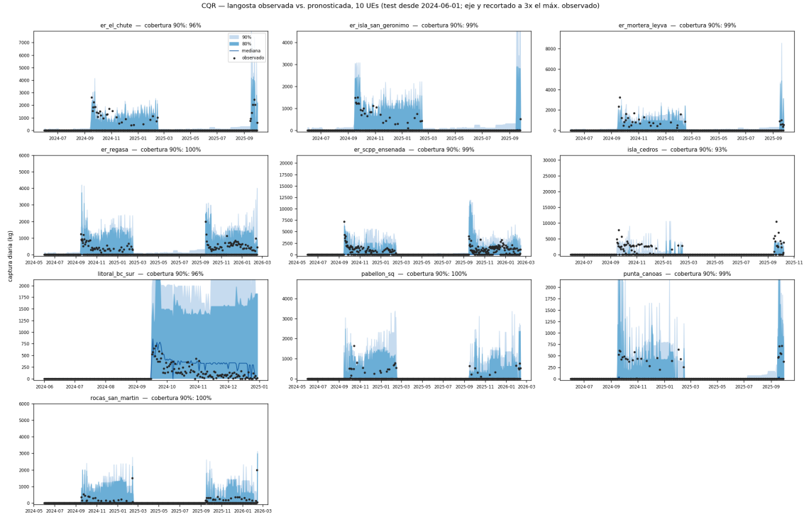
Figure 6: Intervalos de la CQR (bandas 80% y 90% + mediana) frente al observado (puntos) para las diez series de langosta, en el corte 01-junio-2024. Con el bache post-ola-de-calor dentro del entrenamiento y la calibración, el observado cae dentro de las bandas de forma consistente (cobertura empírica anotada por panel, 93–100%), incluida la langosta de San Quintín (96.2%). El eje y de cada panel se recorta a 3\times su máximo observado, pues la cota superior del 90% se dispara en los días pico al invertir la transformación logarítmica.
