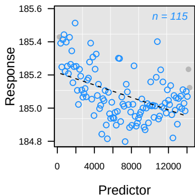
-- L pc Rank 1: y = 185.21 - 0.0000 \cdot x
