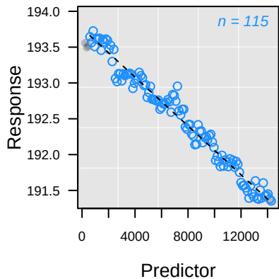
-- L pc Rank 1: y = 193.76 - 0.0002 \cdot x
