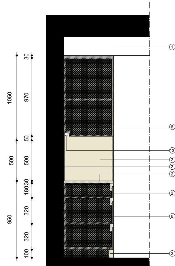
doorsnede D-1.2
