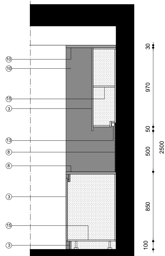
doorsnede D-1.3
