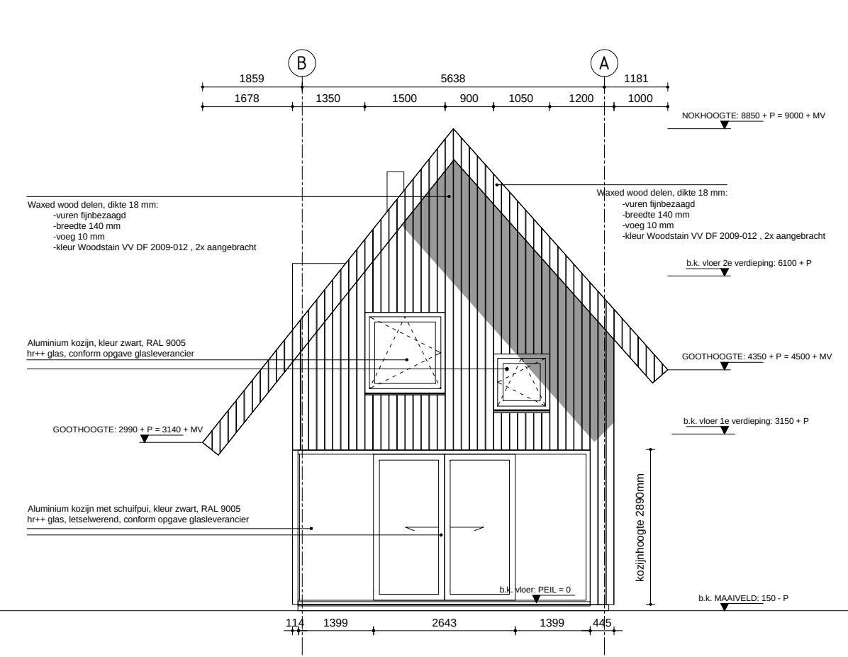
AANZICHT WESTGEVEL (SCHAAL 1:100)
