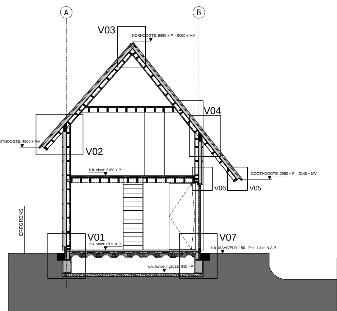
DRSN AA (SCHAAL 1:100)
