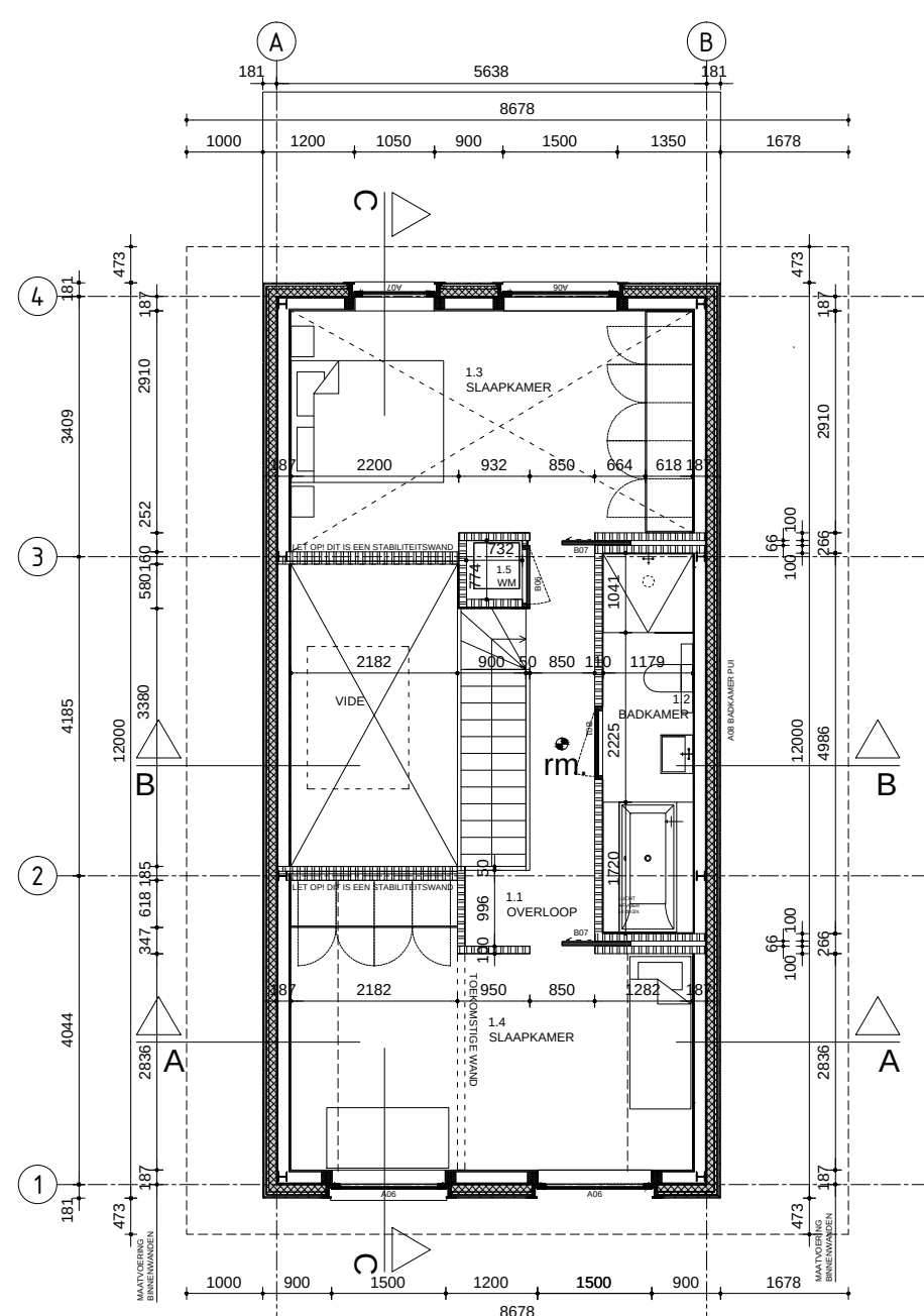
1e VERDIEPING (SCHAAL 1:100)
