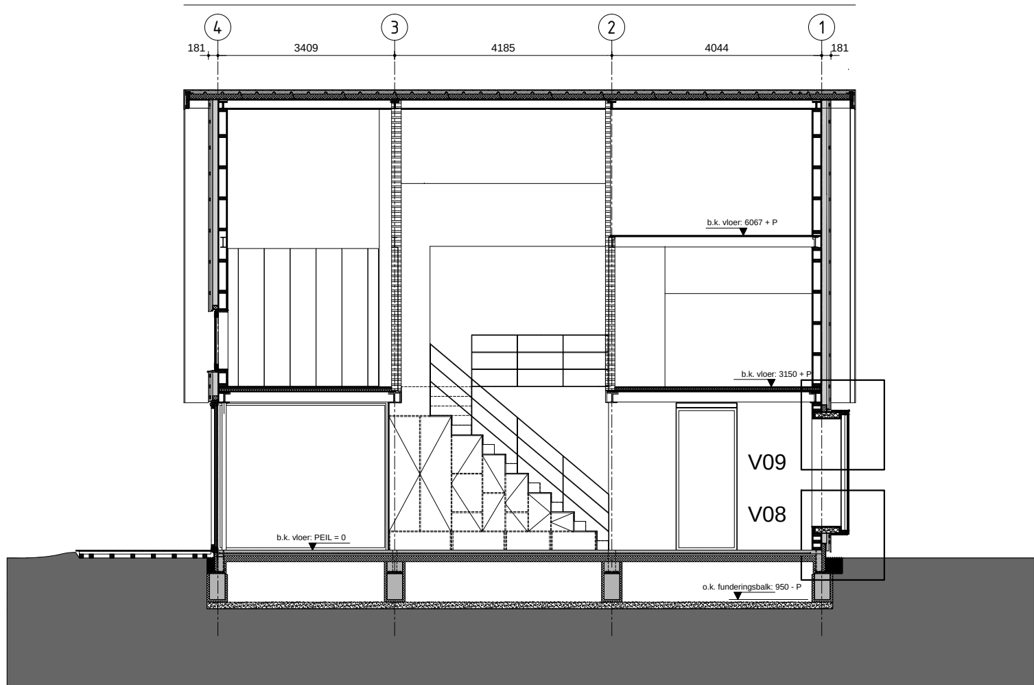
DRSN CC (SCHAAL 1:100)
