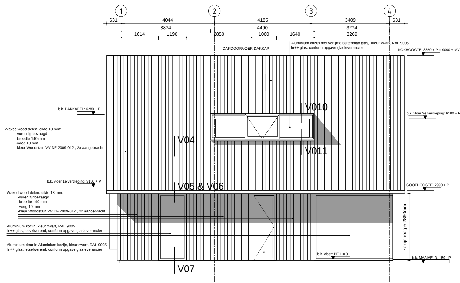
AANZICHT NOORDGEVEL (SCHAAL 1:100)
