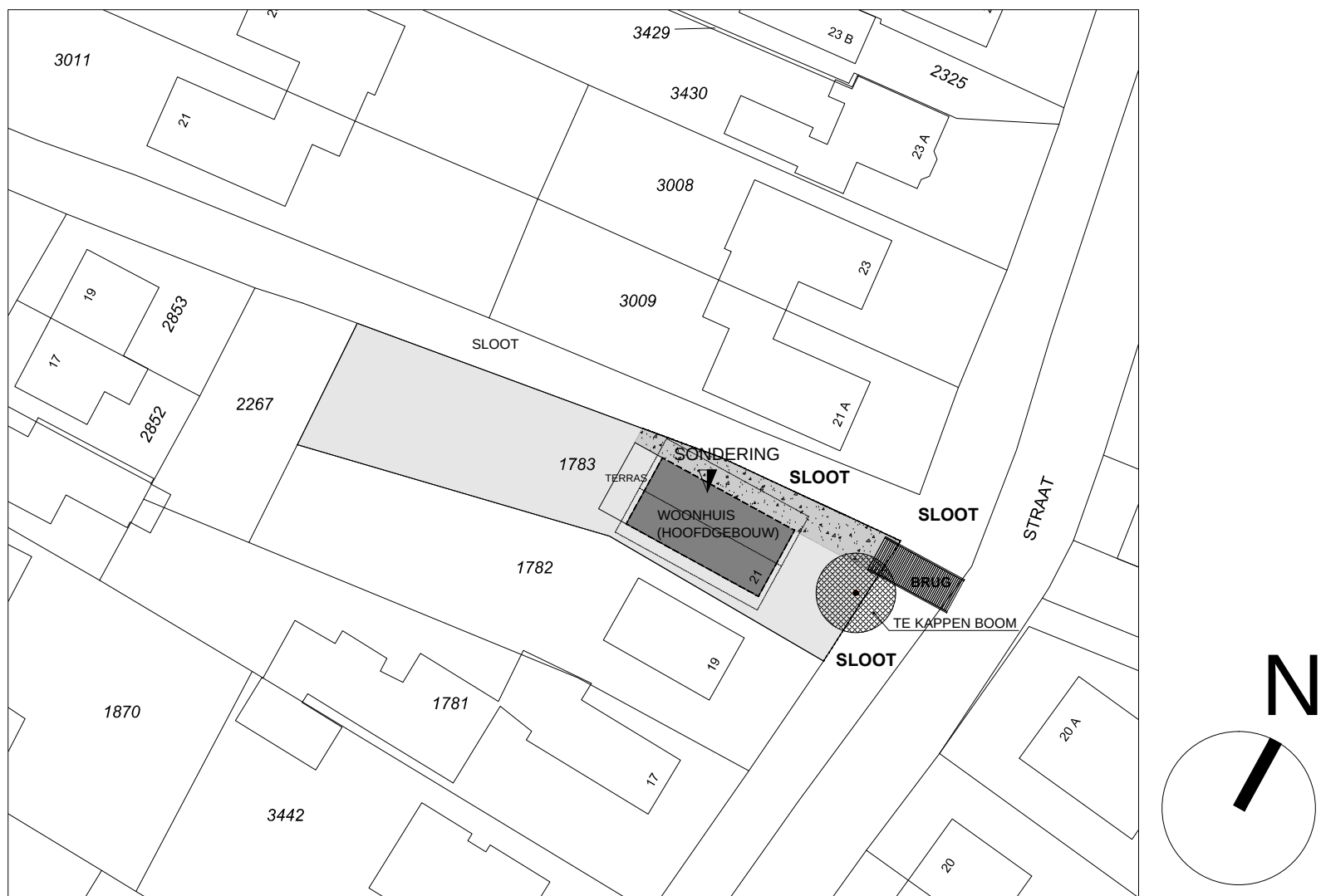
SITUATIE (SCHAAL 1:500)
