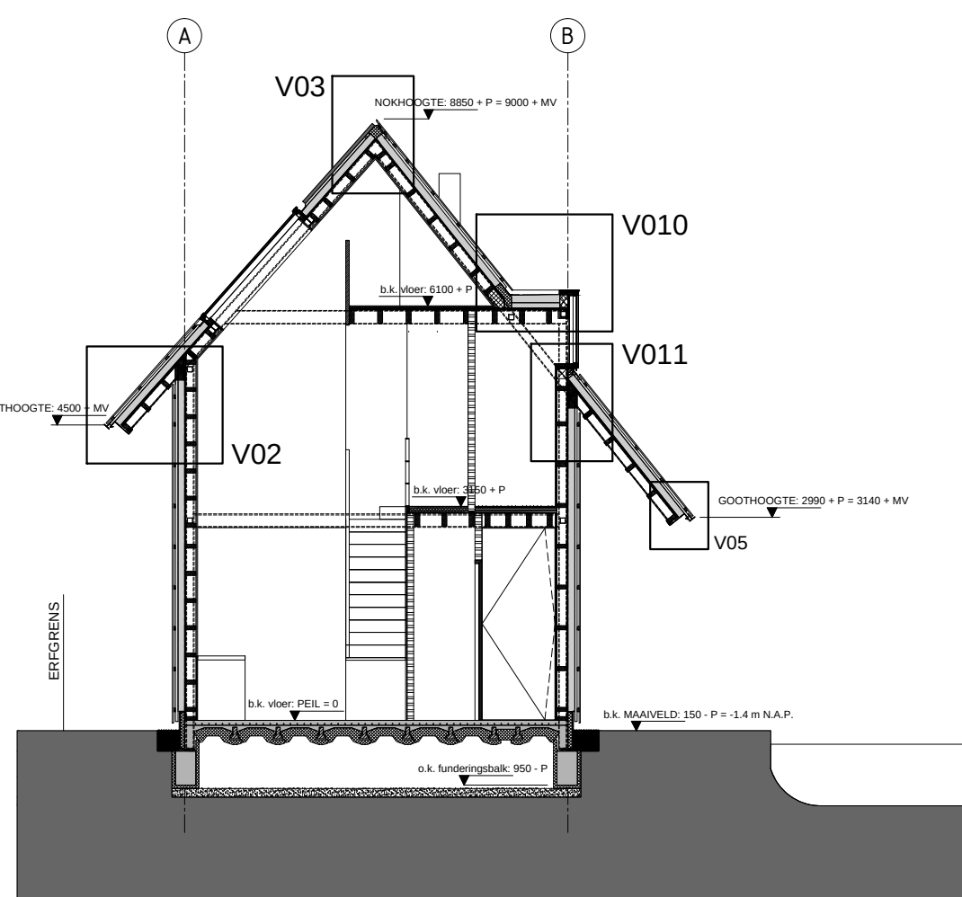
DRSN BB (SCHAAL 1:100)
