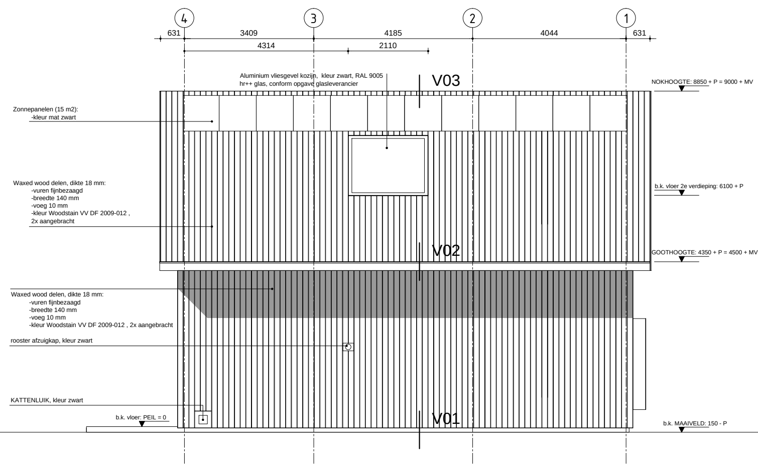
AANZICHT ZUIDGEVEL (SCHAAL 1:100)
