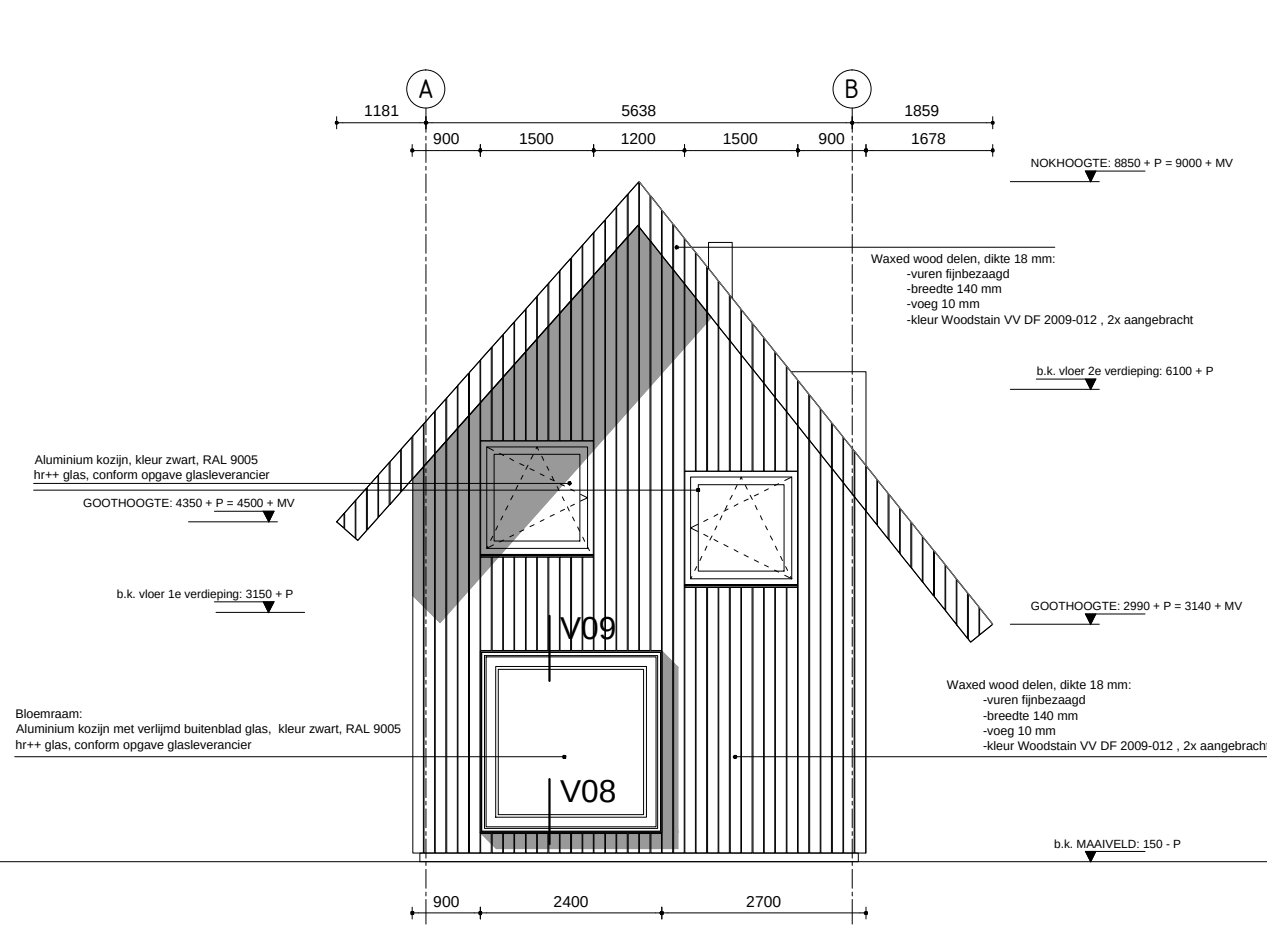
AANZICHT OOSTGEVEL (SCHAAL 1:100)
