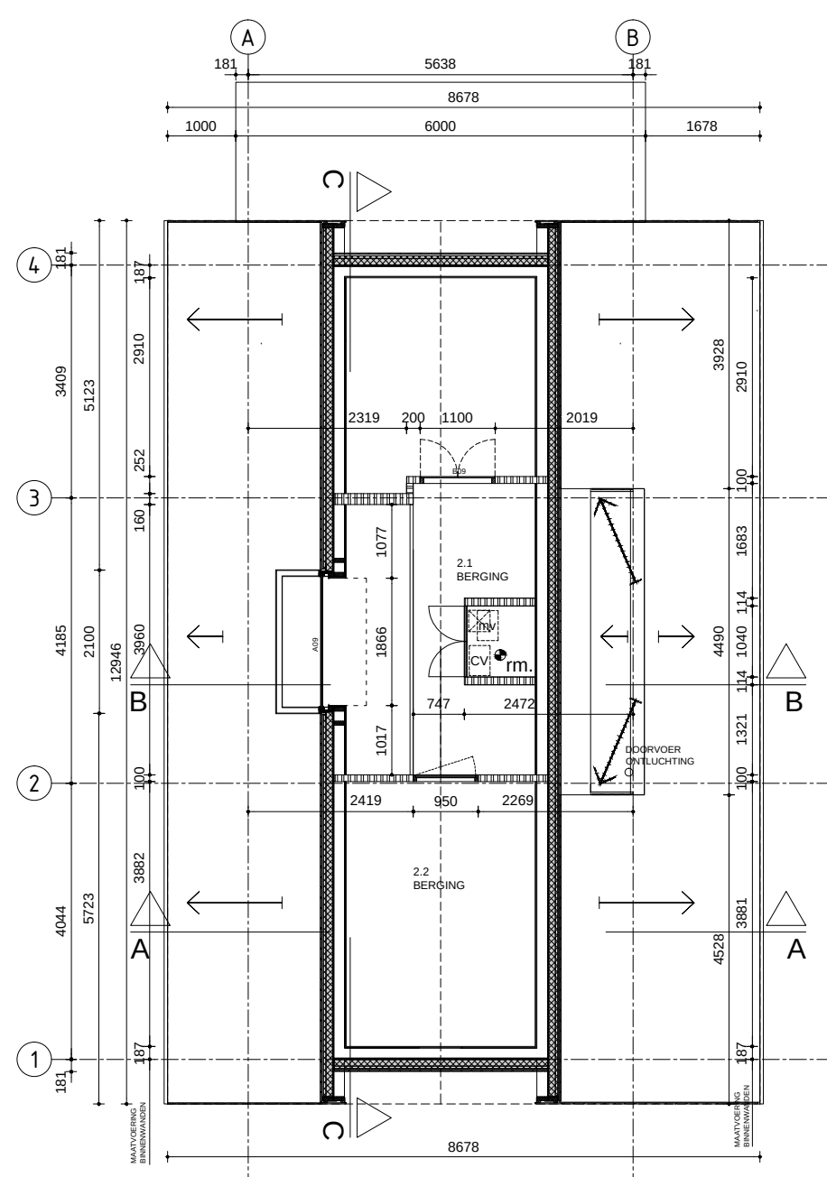
KAPVERDIEPING (SCHAAL 1:100)
