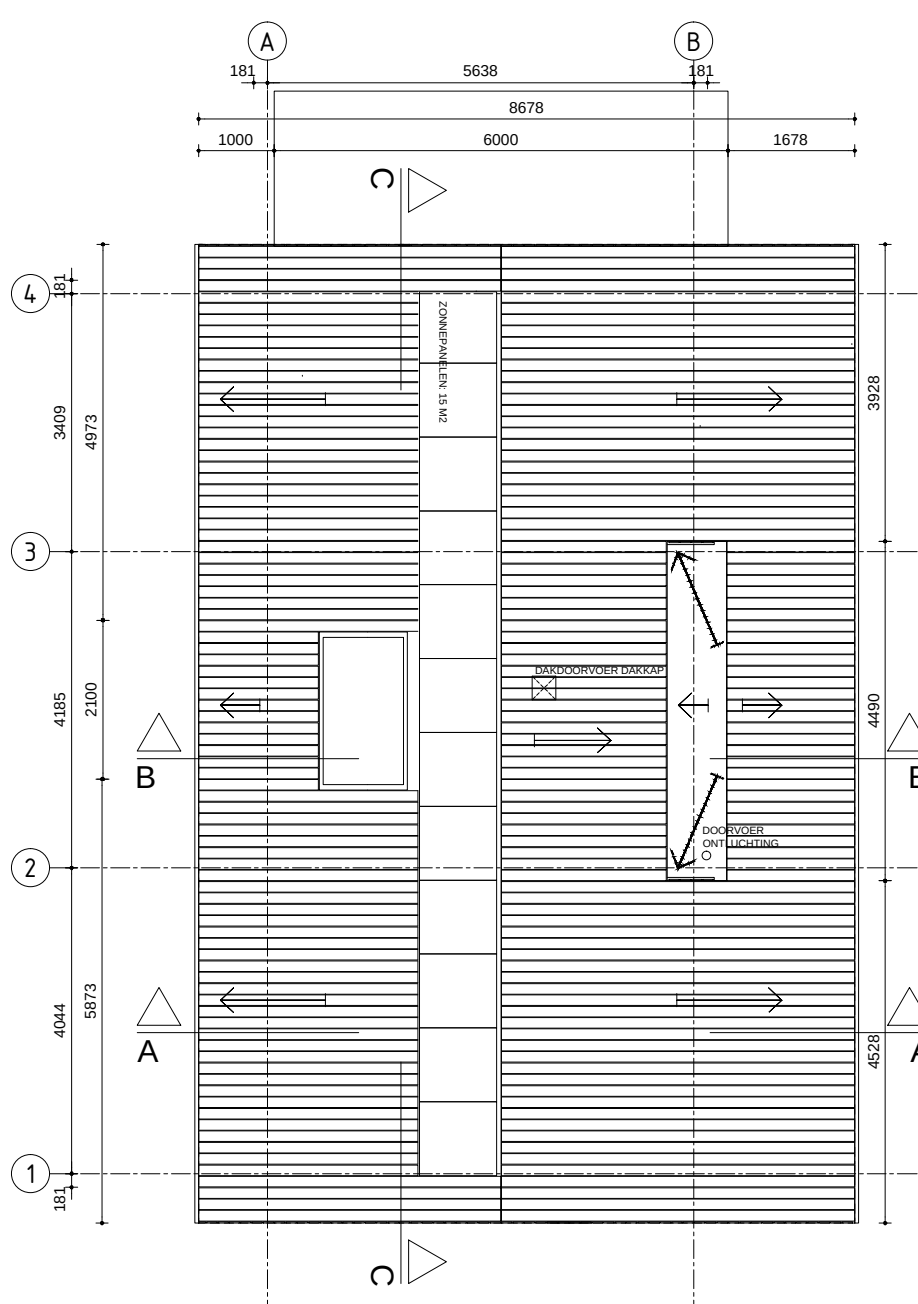
KAPAANZICHT (SCHAAL 1:100)
