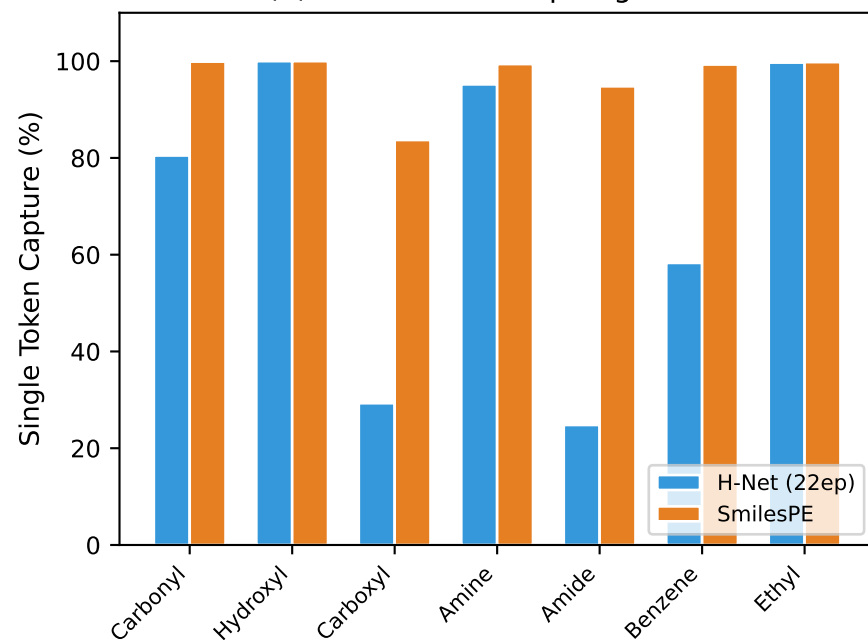
(d) Functional Group Alignment
