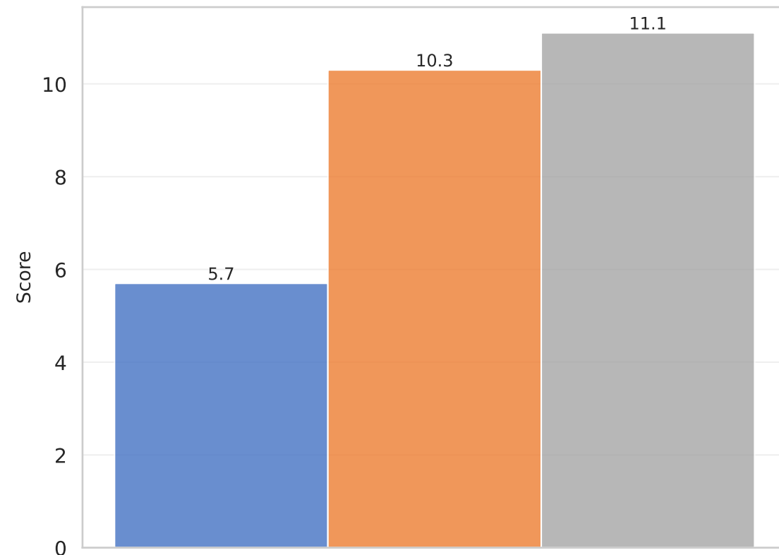
MAC (MAE)
