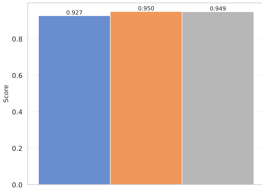
BBBP (AUC)
