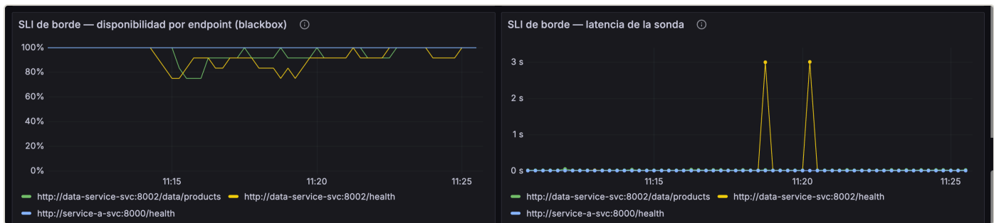
Figura 12. El SLI de borde durante la corrida A. Caen sondas de /data/products y las de /health , mientras service-a /health , fuera del blast radius, permanece en el 100 %. Cada caída de /health es un fallo que el kubelet contabiliza para matar el contenedor: la causa del crash-loop, medida desde fuera. Los picos de 3 s en el panel derecho son sondas agotando el timeout del exporter.
