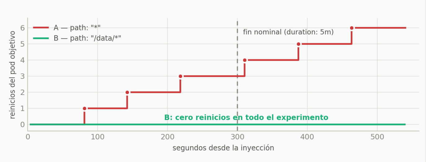
Figura 12. Reinicios acumulados del pod seleccionado.
