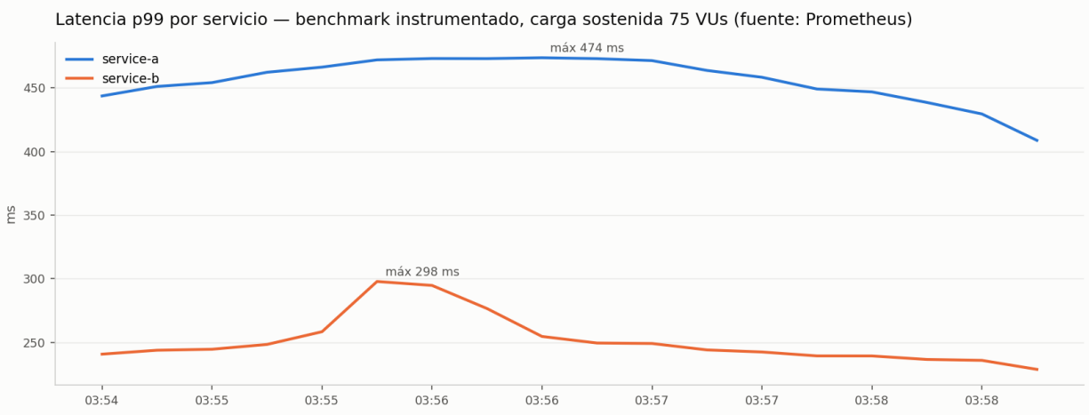
Fig. 3 — Latencia p99 por servicio durante el benchmark (datos reales consultados a Prometheus).
