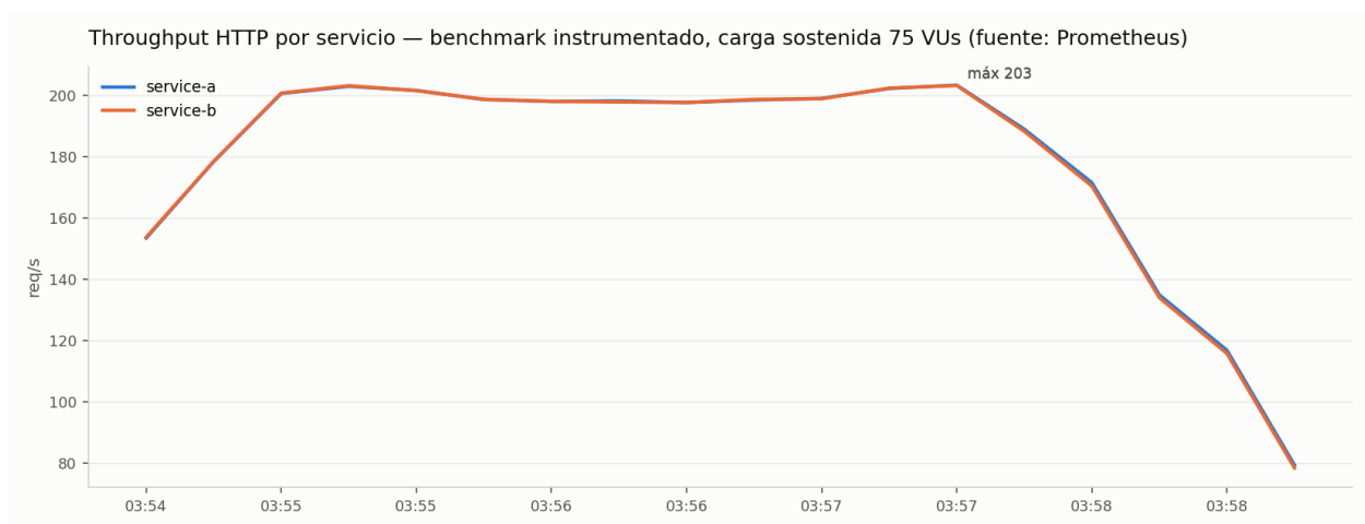
Fig. 4 — Throughput por servicio en la misma ventana; service-b recibe una llamada por cada orden de service-a.
