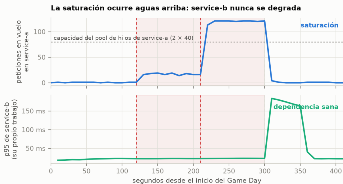
Figura 2. Experimento 1, señales de Prometheus. Arriba, las peticiones en vuelo en service-a llegan a 121, por encima de las 80 ranuras de su pool de hilos: la cola es lo que amplifica el retardo. Abajo, el p95 propio de service-b se mantiene en 22-23 ms durante toda la inyección. Un tablero centrado en la dependencia habría permanecido en verde durante todo el incidente.
