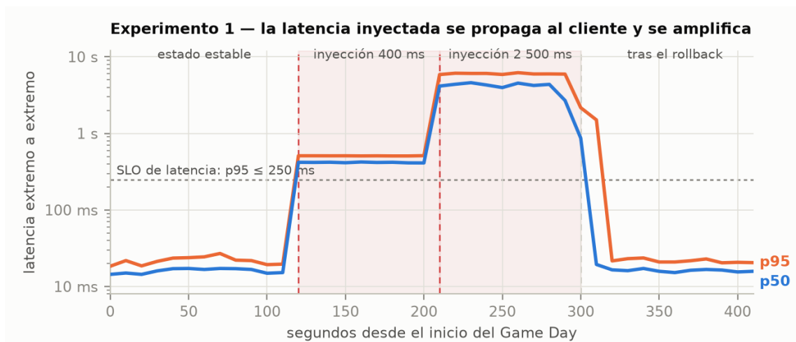
Figura 1. Experimento 1. La latencia inyectada (bandas sombreadas) atraviesa el sistema sin amortiguación alguna: el p50 pasa de 16,0 ms a 417,4 ms con 400 ms inyectados —propagación 1:1— y a 4 153,5 ms con 2 500 ms inyectados, es decir 1,66 \times el retardo inyectado. Escala logarítmica. Elaboración propia a partir de 16 800 peticiones medidas en el cliente.
