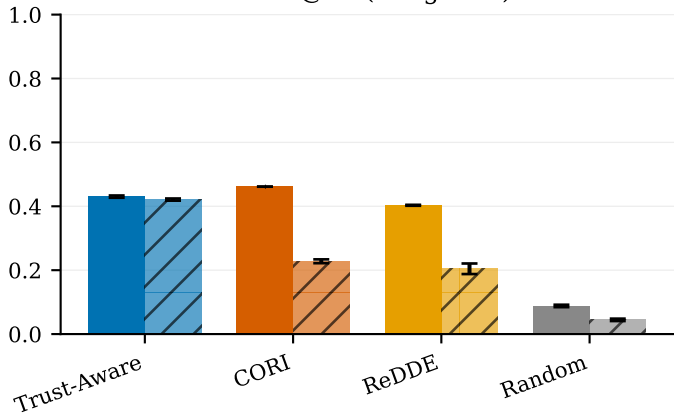
nDCG@10 (budget=1)
