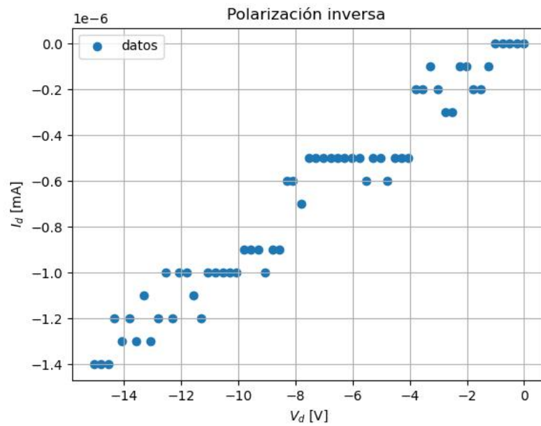
Figura 4. Corriente sobre diodo en polarización inversa, variando el voltaje de 0V a 15V en pasos de 0.5V, a una temperatura de 24°C.
