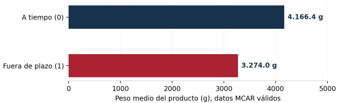
Figura 2. Comparación de pesos medios con datos válidos de la versión MCAR (n = 9.899).
