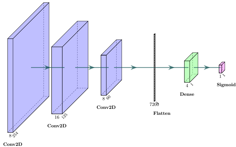
Figura 2.5: Arquitectura CNN-CT-Drop . Tres capas Conv2D (8, 16 y 8 filtros) con Dropout del 50 % tras cada bloque para regularización. La resolución se reduce de 254x254 a 30x30, generando un vector aplanado de 7.200 valores conectado a una capa Dense de 4 neuronas y salida Sigmoid.
