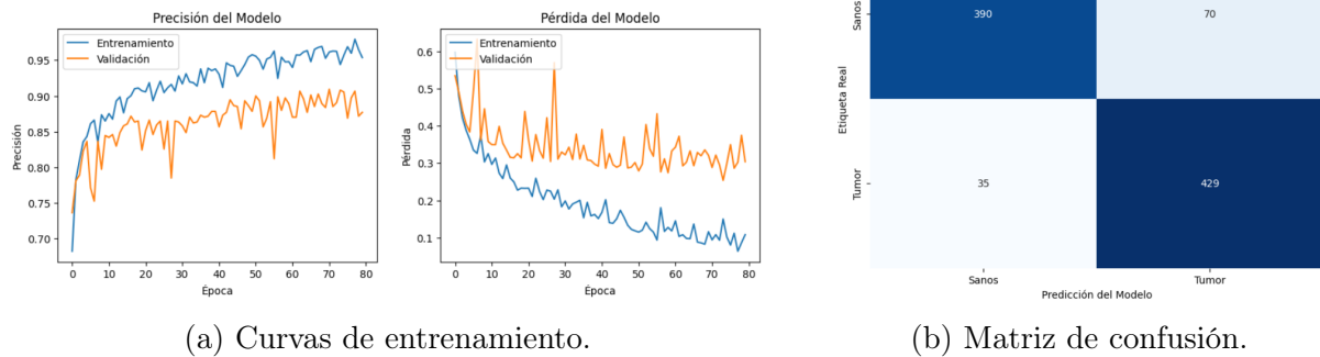
Figura 3.11: Resultados del modelo ResNet50-TL-CT sobre el conjunto de CT. Mejora notablemente respecto al FT, pero al final las curvas divergen indicando inicio de sobreajuste. Alcanza un 88.64 % de accuracy (390 VN, 429 VP, 70 FP, 35 FN), limitado por entrenar solo la parte final.
