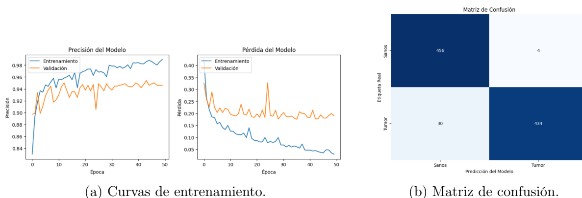
Figura 3.6: Resultados del modelo VGG16-TL-CT sobre el conjunto de CT. Presenta sobreajuste notable al entrenar solo la parte final de la red, lo que sugiere que el clasificador memoriza patrones sin generalizar. Aun así obtiene un 96.32 % de accuracy (456 VN, 434 VP, 4 FP, 30 FN).
