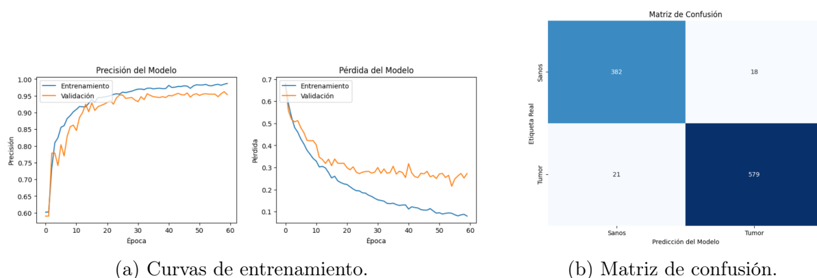
Figura 3.16: Resultados del modelo CNN-MRI-Drop sobre el conjunto de MRI. Las curvas mejoran respecto al modelo base, aunque aparece cierto sobreajuste en la pérdida al final. Gran salto en rendimiento con un 96 % de accuracy (382 VN, 579 VP, 18 FP, 21 FN).
