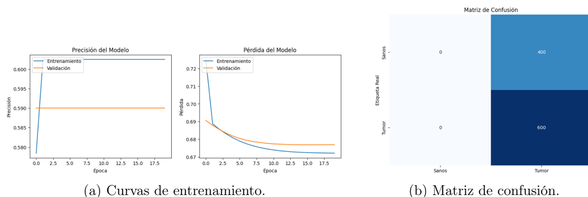
Figura 3.15: Resultados del modelo CNN-MRI-Base sobre el conjunto de MRI. Las curvas de accuracy son planas con gran separación entre entrenamiento y validación. La matriz revela que el modelo clasifica todas las imágenes como tumor (0 VN, 600 VP, 400 FP, 0 FN), obteniendo solo un 60 % de accuracy.
