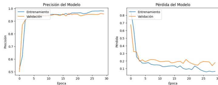
Figura 3.9: Curvas de entrenamiento de la primera solución propuesta con el modelo VGG16 para el conjunto de CT.
