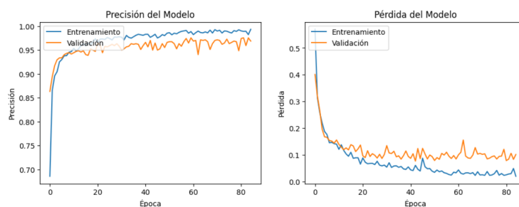
Figura 3.5: Curvas de entrenamiento del tercer modelo creado para el conjunto de CT.
