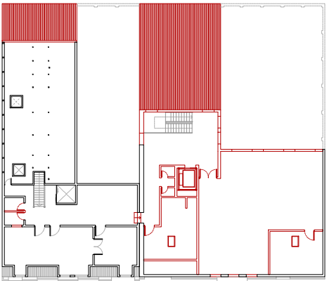
Planta Segunda
