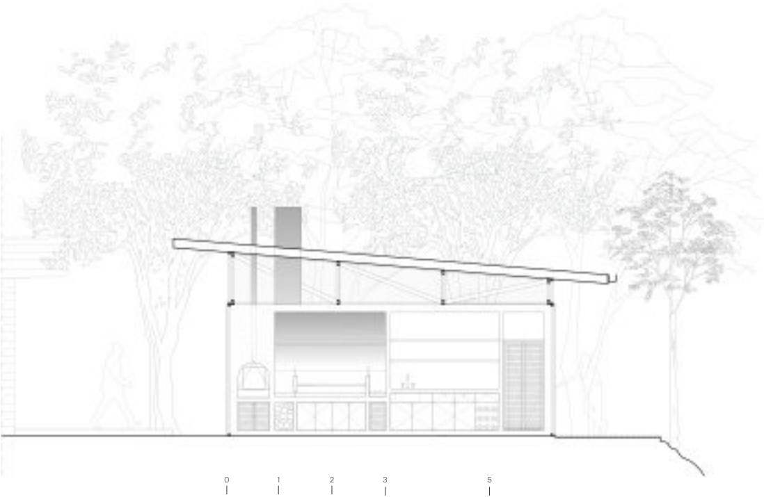
Sección
