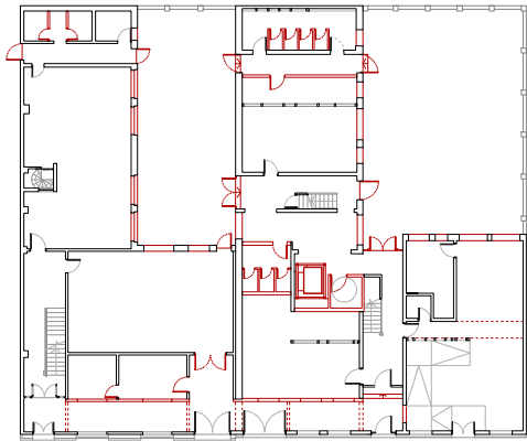
Planta Baja
