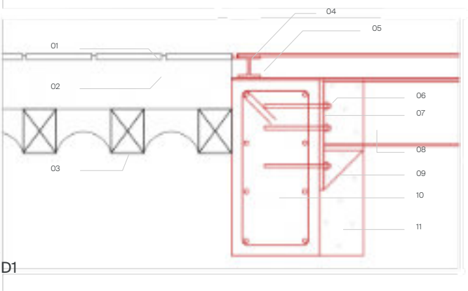
Detalles
