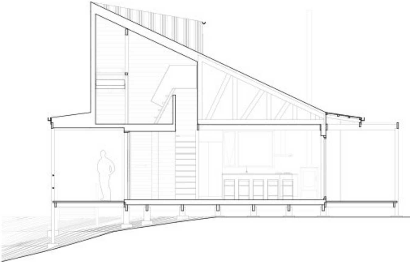
Sección
