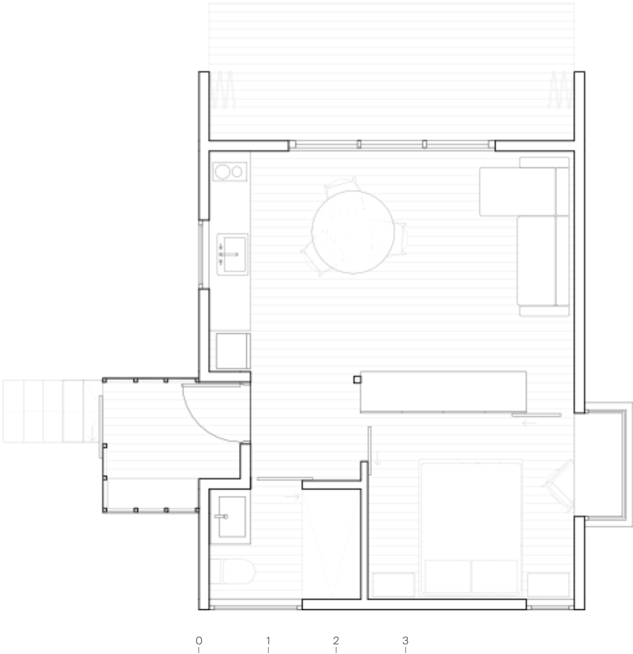
Planta Baja
