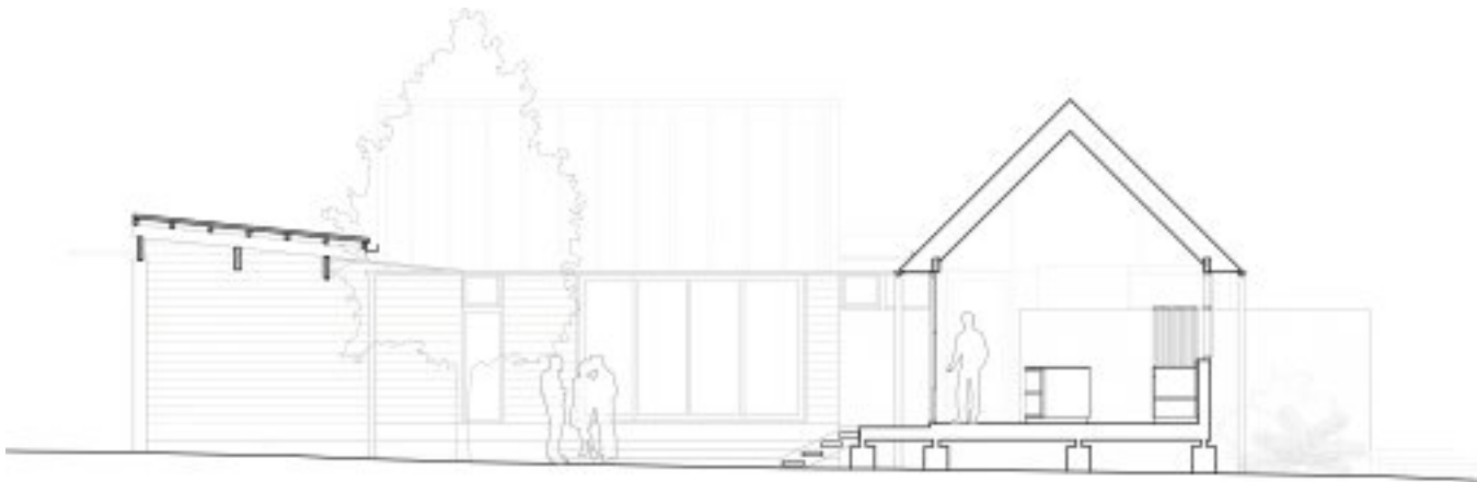
Sección
