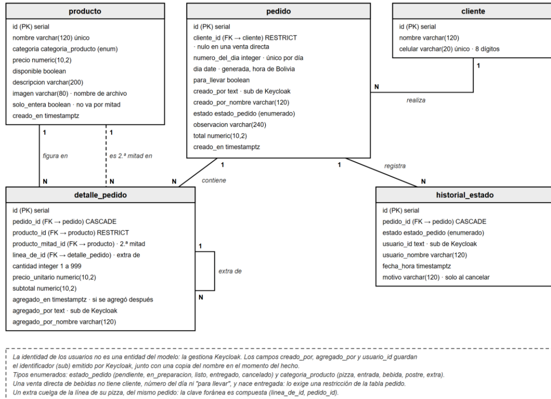
Figura 4. Modelo entidad-relación. Fuente: elaboración propia.
