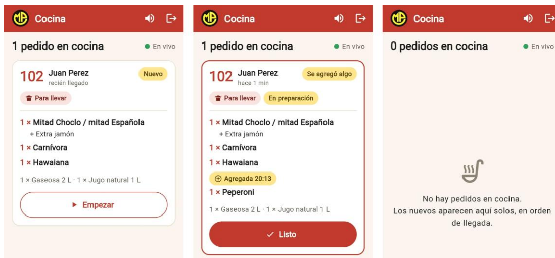
Figura 8. Cola de cocina en un celular: el pedido recién llegado (izquierda), en preparación y con una pizza agregada por recepción (centro), y la cola vacía después de marcarlo como listo (derecha). Fuente: captura del sistema desplegado, 25/09/2026.
