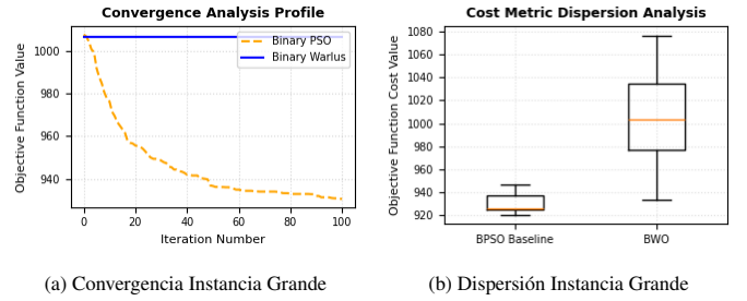
Figura 3: Trayectorias de convergencia y diagramas de caja para la instancia grande ( 20 \times 50 ), mostrando la explotación local efectiva de BPSO y la explotación extendida de BWO.
