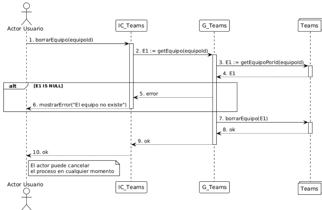
Figura 53. Diagrama de Secuencia de CU009. Borrado de equipos.
