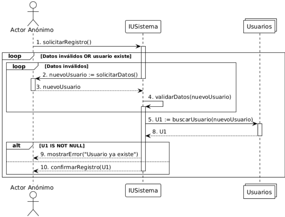
Figura 15. Diagrama de Secuencia de CU001. Registro de usuario.
