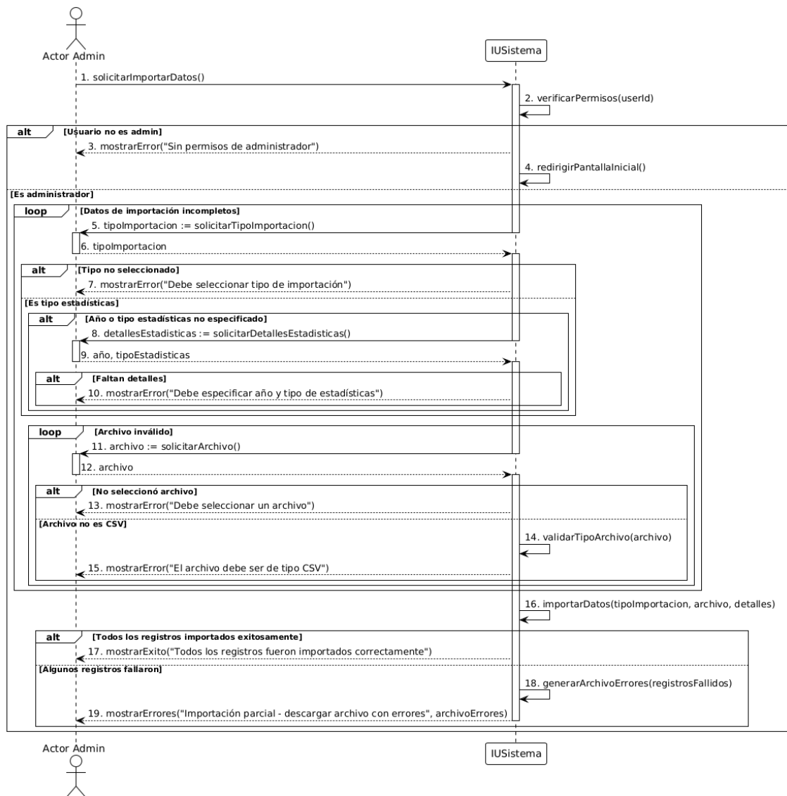
Figura 31. Diagrama de Secuencia de CU017. Importación de datos.
