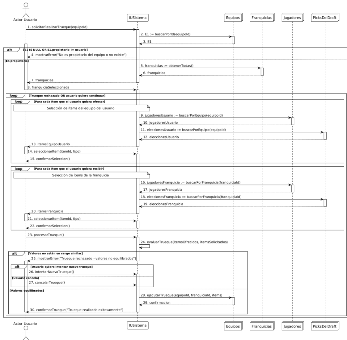
Figura 27. Diagrama de Secuencia de CU013. Realización de trueques.
