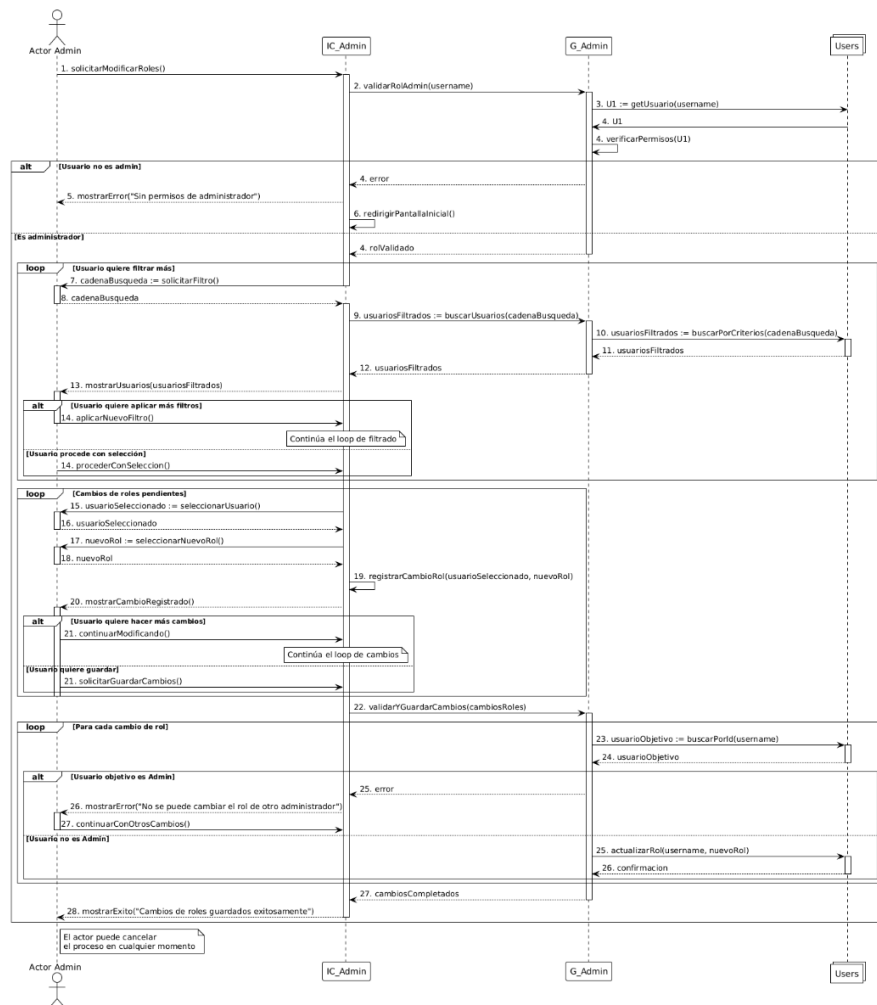
Figura 62. Diagrama de Secuencia de CU018. Alteración de roles de usuarios.
