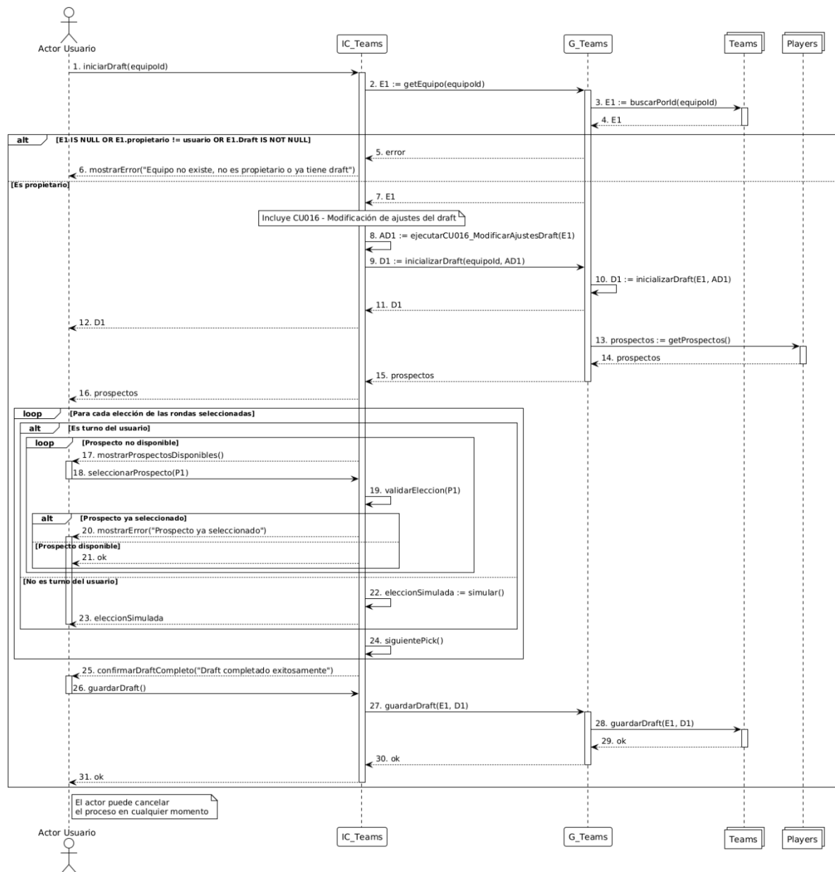
Figura 58. Diagrama de Secuencia de CU014. Realización del draft.
