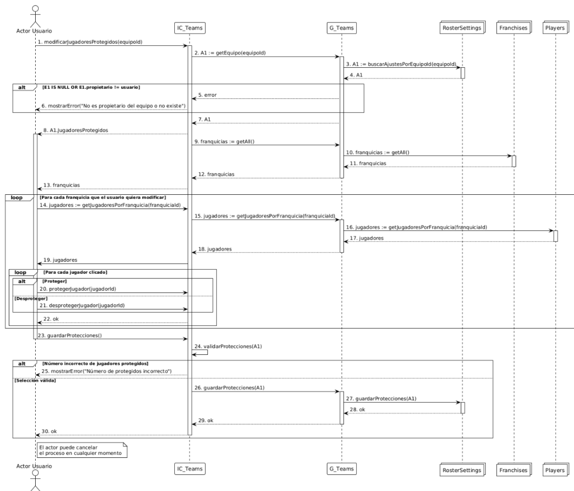
Figura 55. Diagrama de Secuencia de CU011. Elección de jugadores protegidos.
