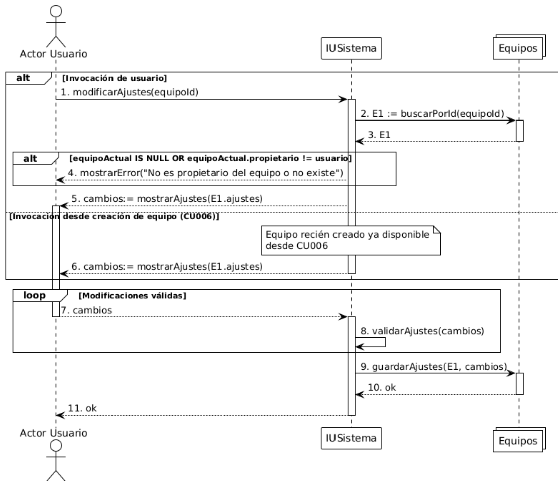
Figura 24. Diagrama de Secuencia de CU010. Modificación de ajustes de juego.
