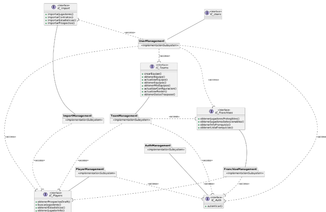
Figura 65. Vista arquitectónica de Implementación
