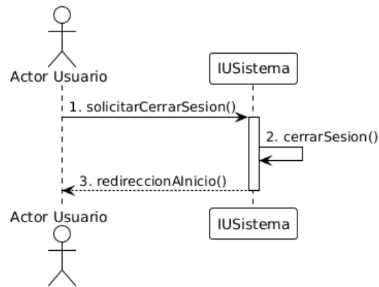
Figura 17. Diagrama de Secuencia de CU003. Cerrado de sesión.
