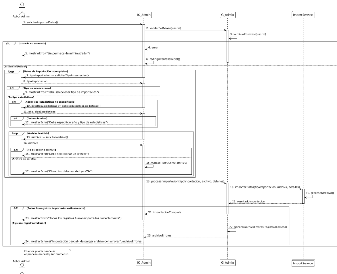
Figura 61. Diagrama de Secuencia de CU017. Importación de datos.
