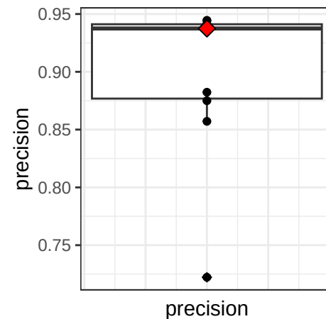
precision (N = 10)
