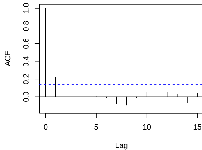
ACF residuales^2 AAPL
