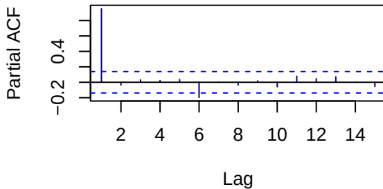
PACF Rendimientos AAPL
