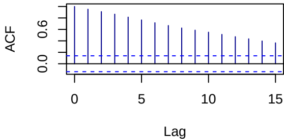
ACF Rendimientos AAPL
