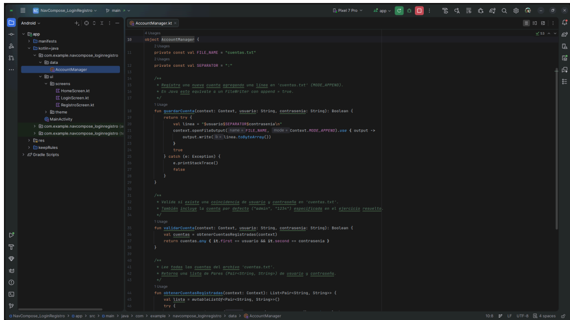
Figura 6: Función guardarCuenta con MODE_APPEND
