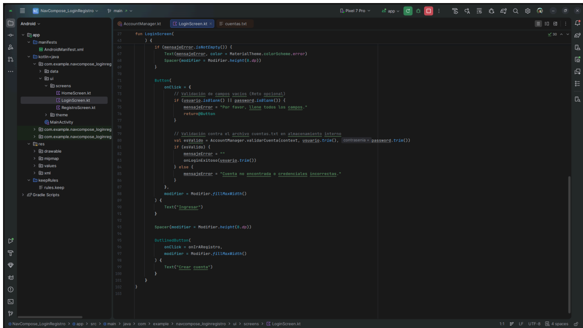
Figura 10: Retorno anticipado ante campos vacíos
