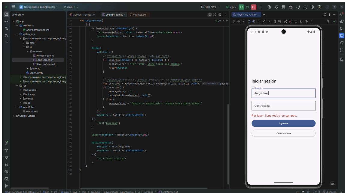
Figura 11: Mensaje de error reactivo en interfaz
