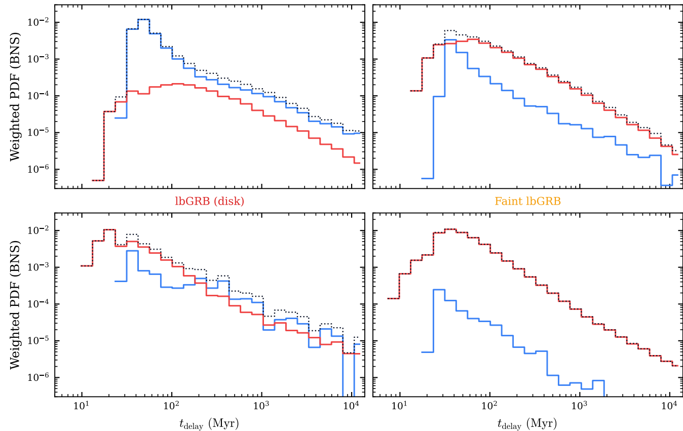
sbGRB + blue KN
