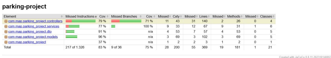
Figura 3 Reporte de cobertura de código JaCoCo — 83%
