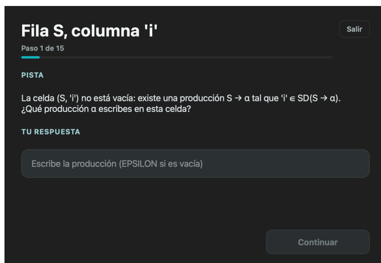
Figura 5 Modo guiado de la tabla LL(1).
