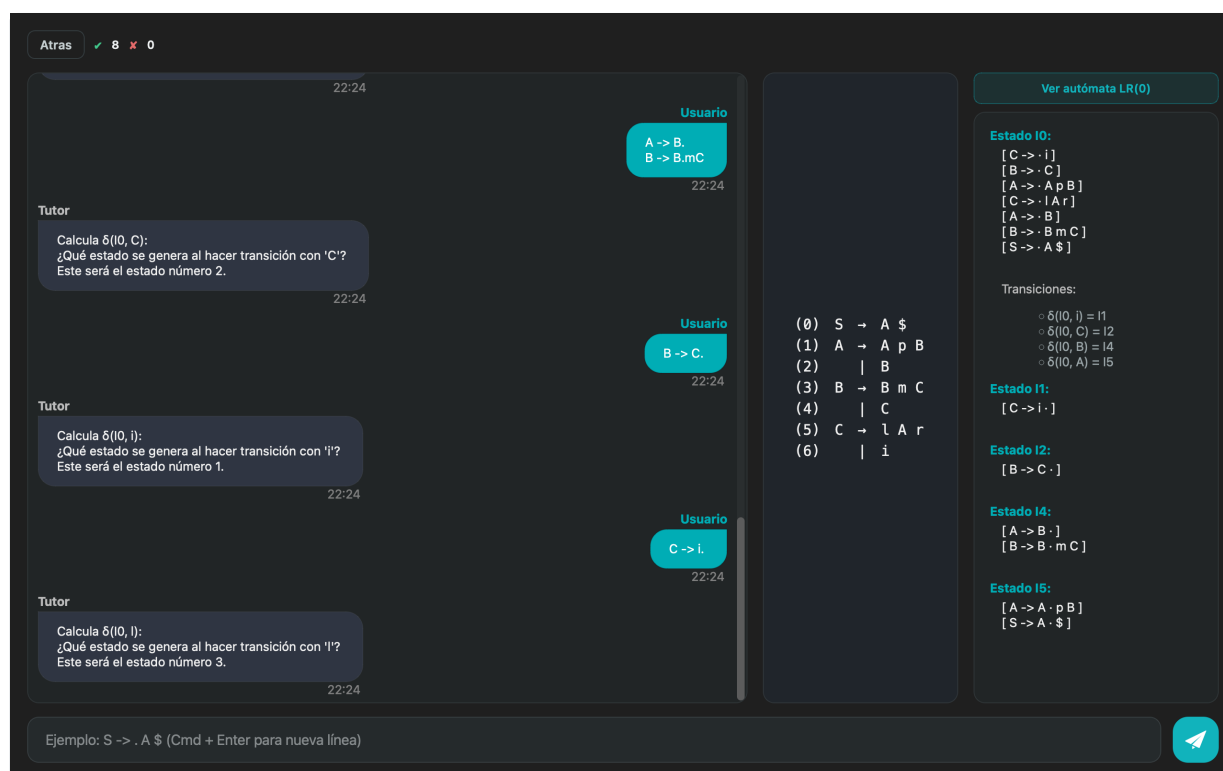
Figura 6 Tutor SLR(1) mientras se calculan las transiciones de un estado. A la derecha, la gramática numerada y los estados construidos.
