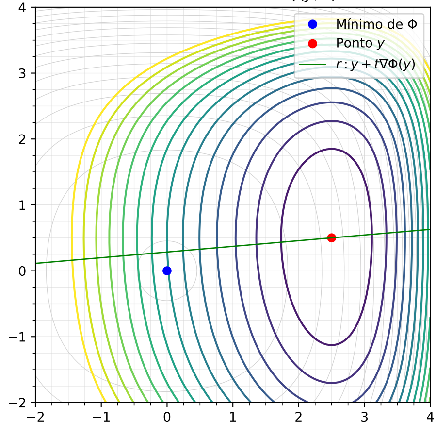
Diferença da seção de \Phi para a reta r
