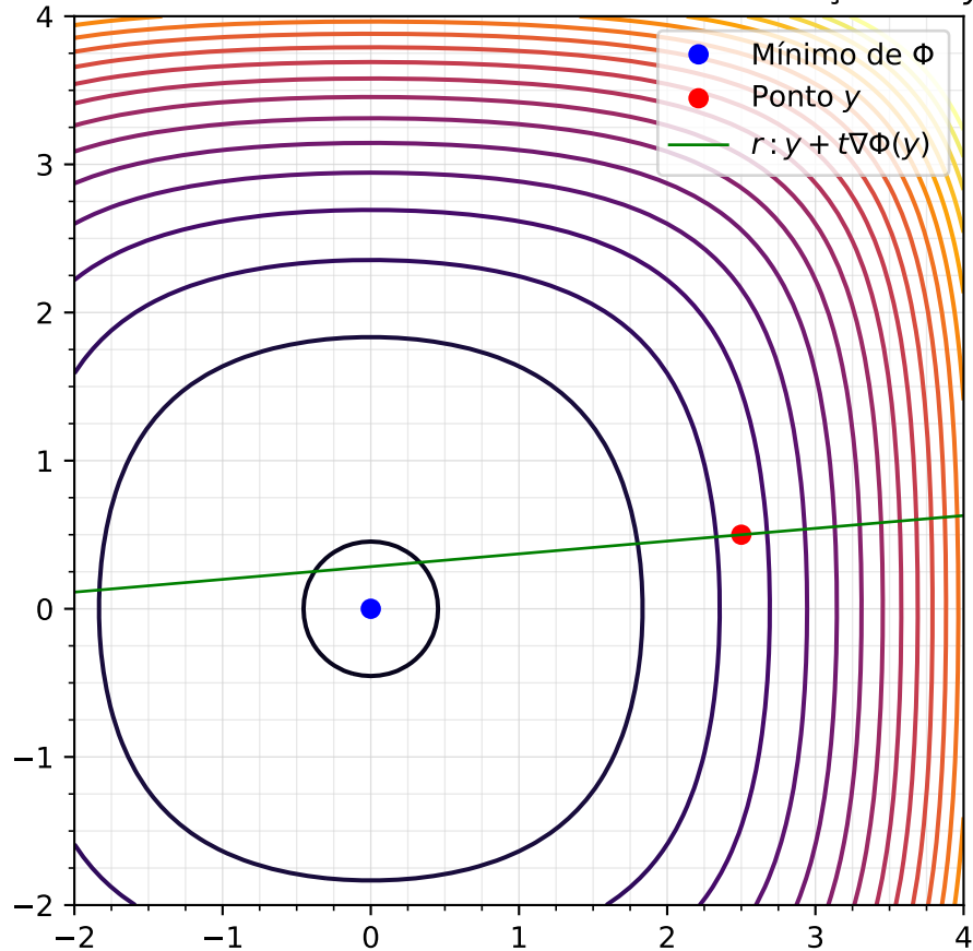
Seção da função \Phi e reta r
