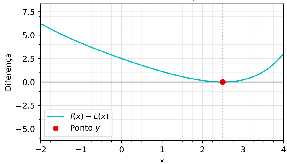
Diferença da seção de \Phi para a reta r
