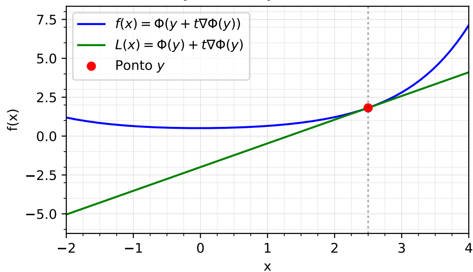
Seção da função \Phi e reta r
