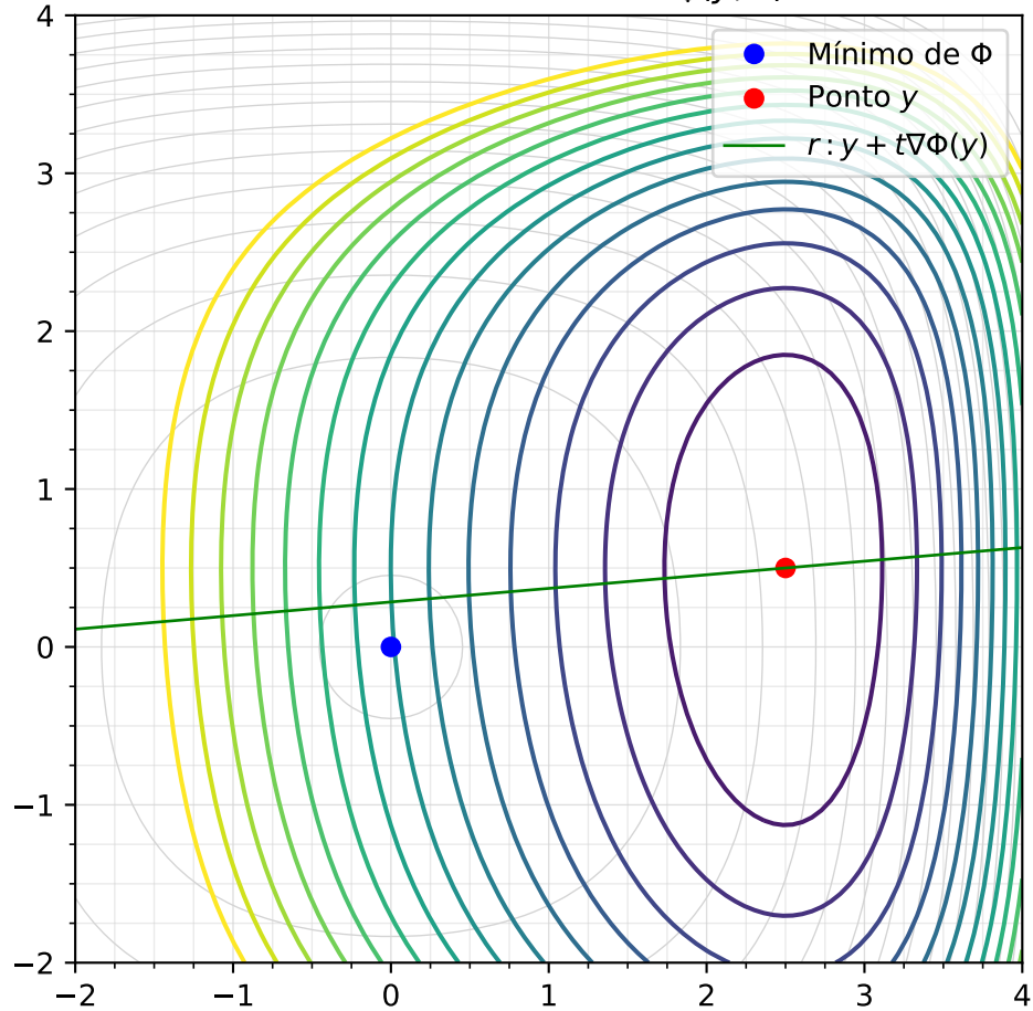
Curvas de nível de D_\Phi(y, x)
