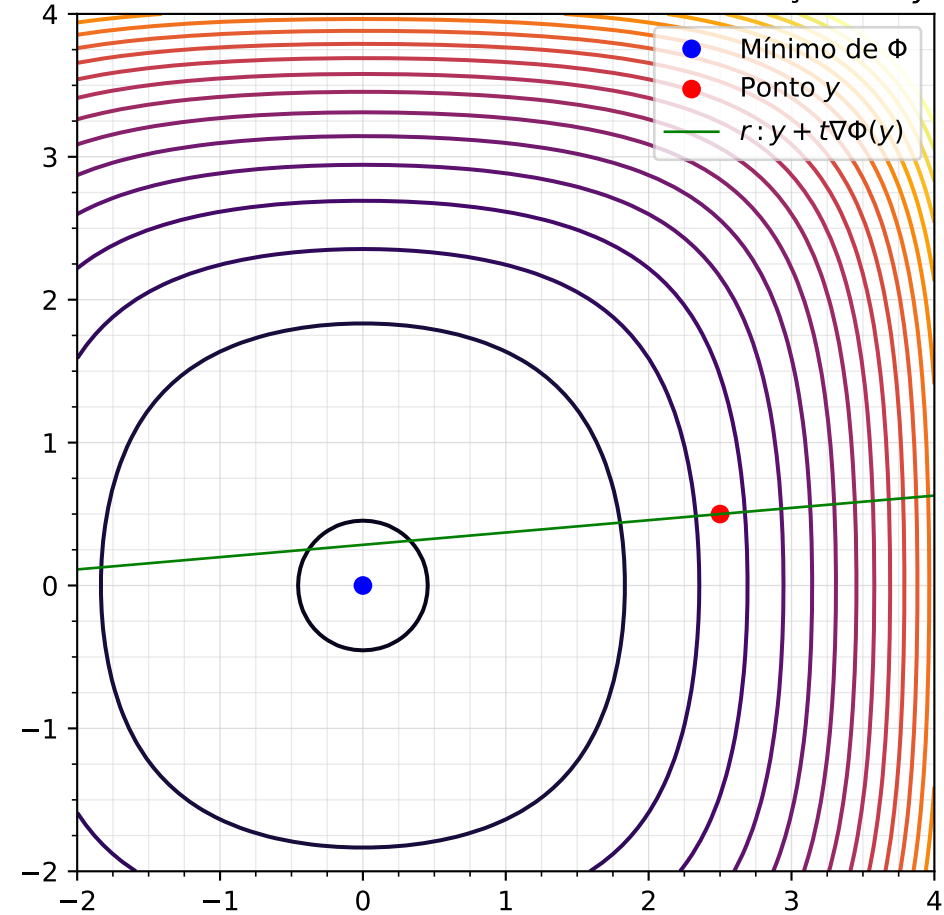
Curvas de nível de \Phi e reta de maior inclinação em y
