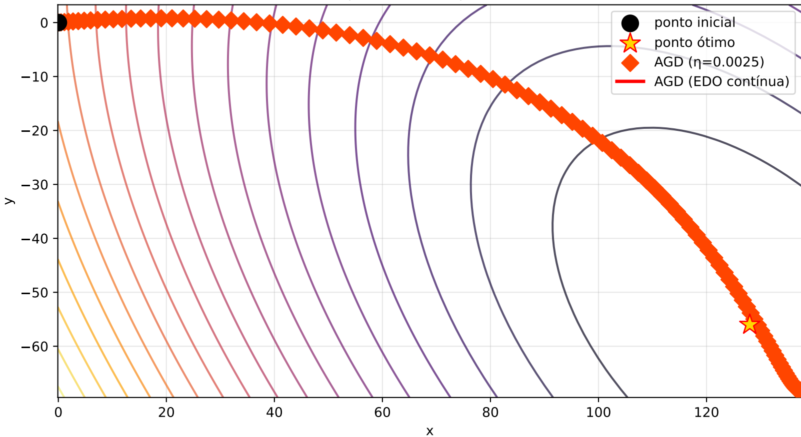
AGD - Espaço Primal ( \eta=0.0025 , T=5 )
