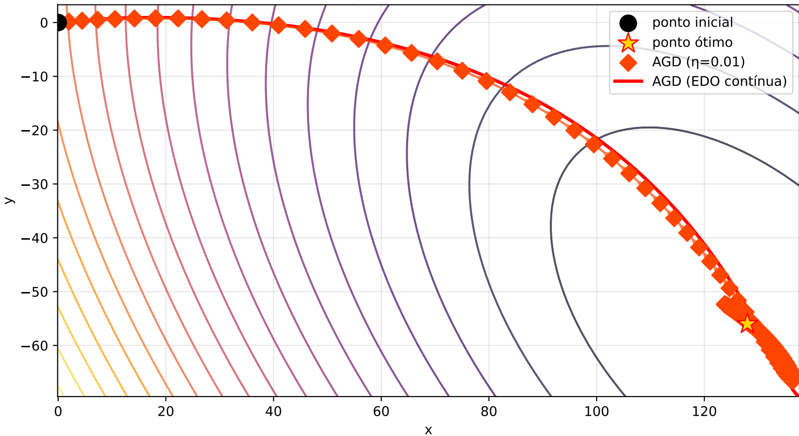
AGD - Espaço Primal ( \eta=0.01 , T=5 )
