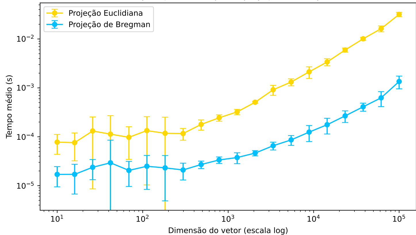
Comparação de tempo de projeção no simplex
