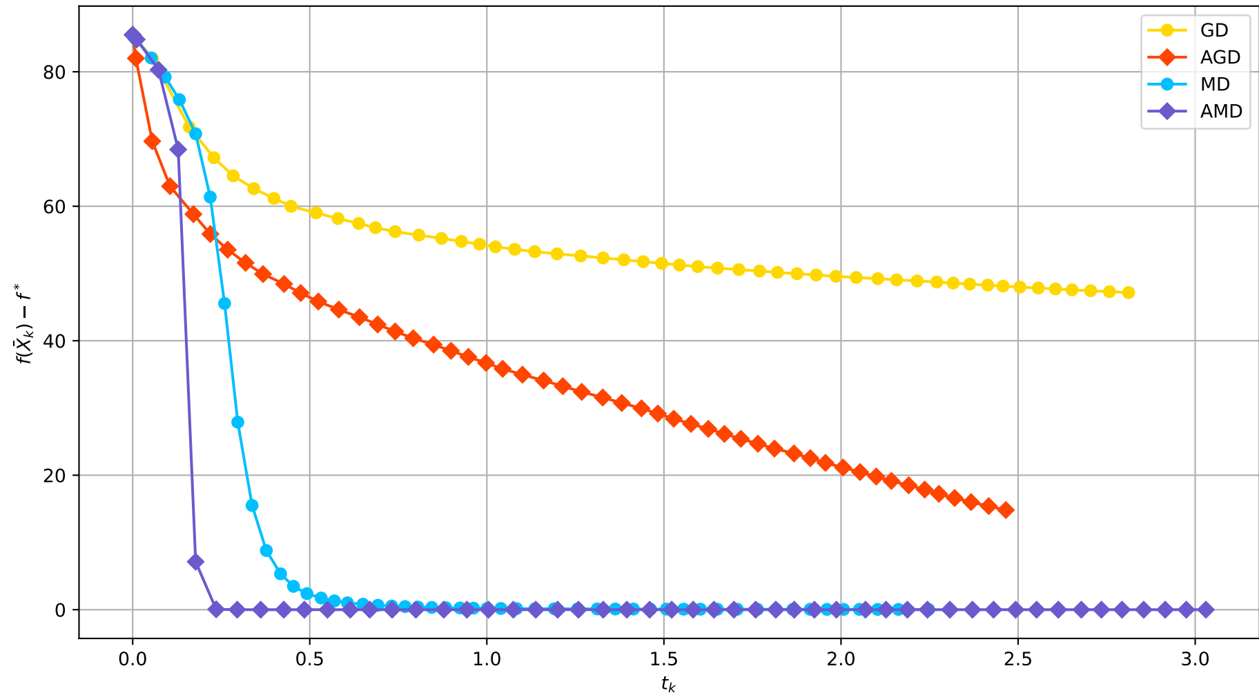
Convergência dos métodos em dimensão 10000
