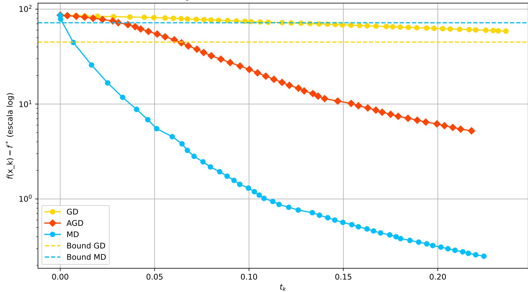
Convergência das médias dos métodos em dimensão 10
