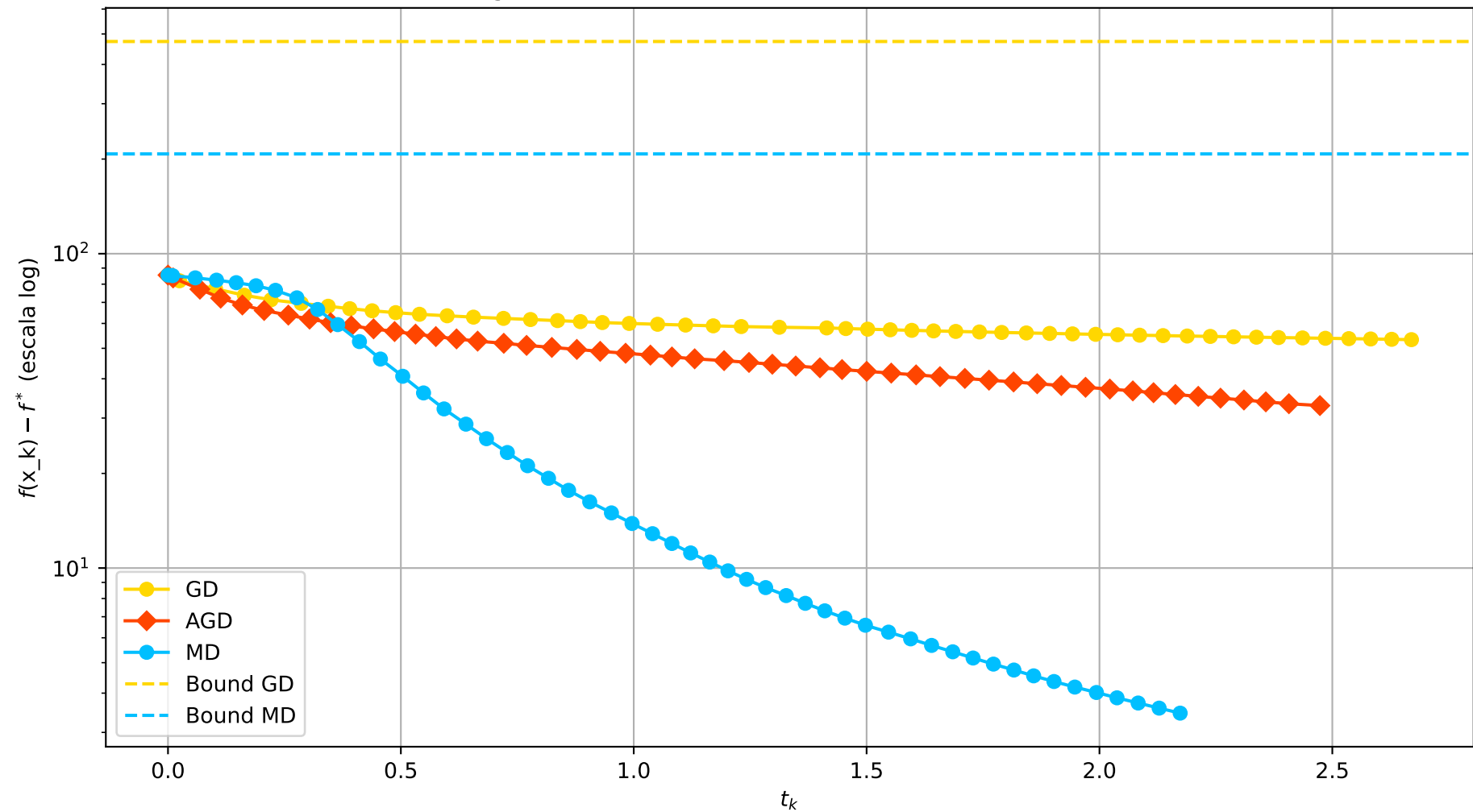
Convergência das médias dos métodos em dimensão 10000
