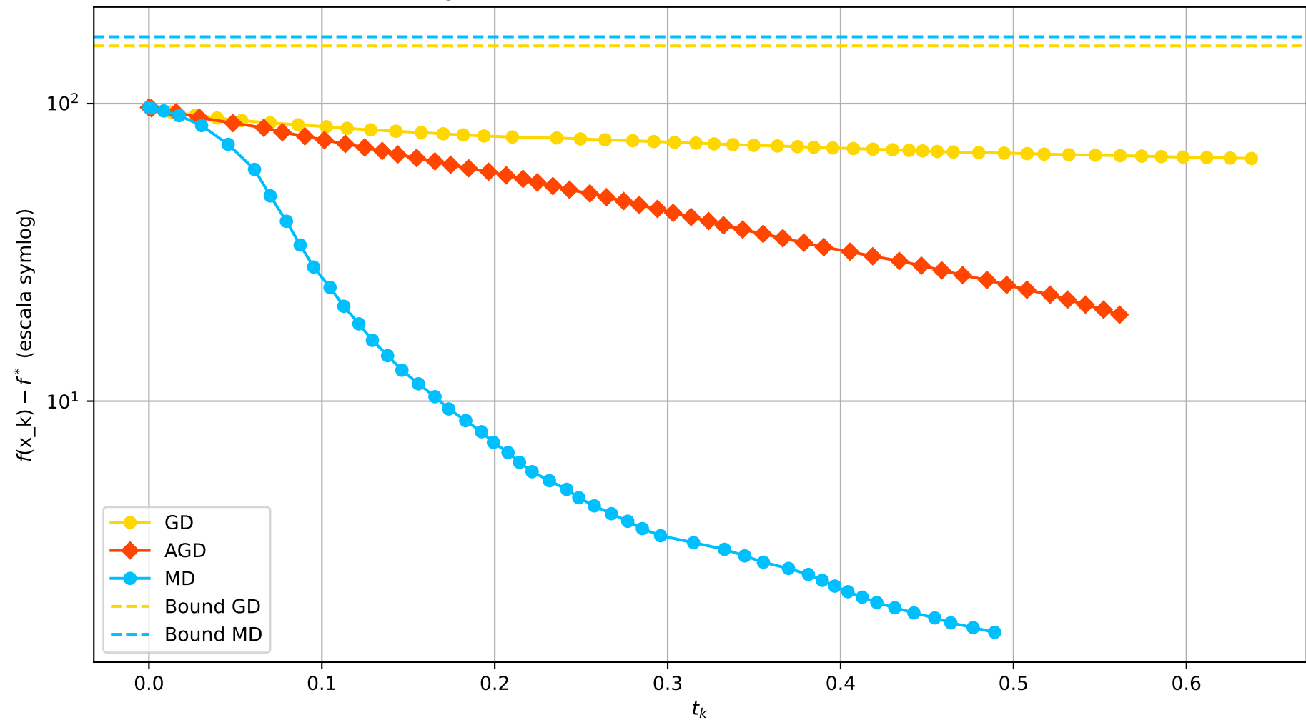
Convergência das médias dos métodos em dimensão 1000
