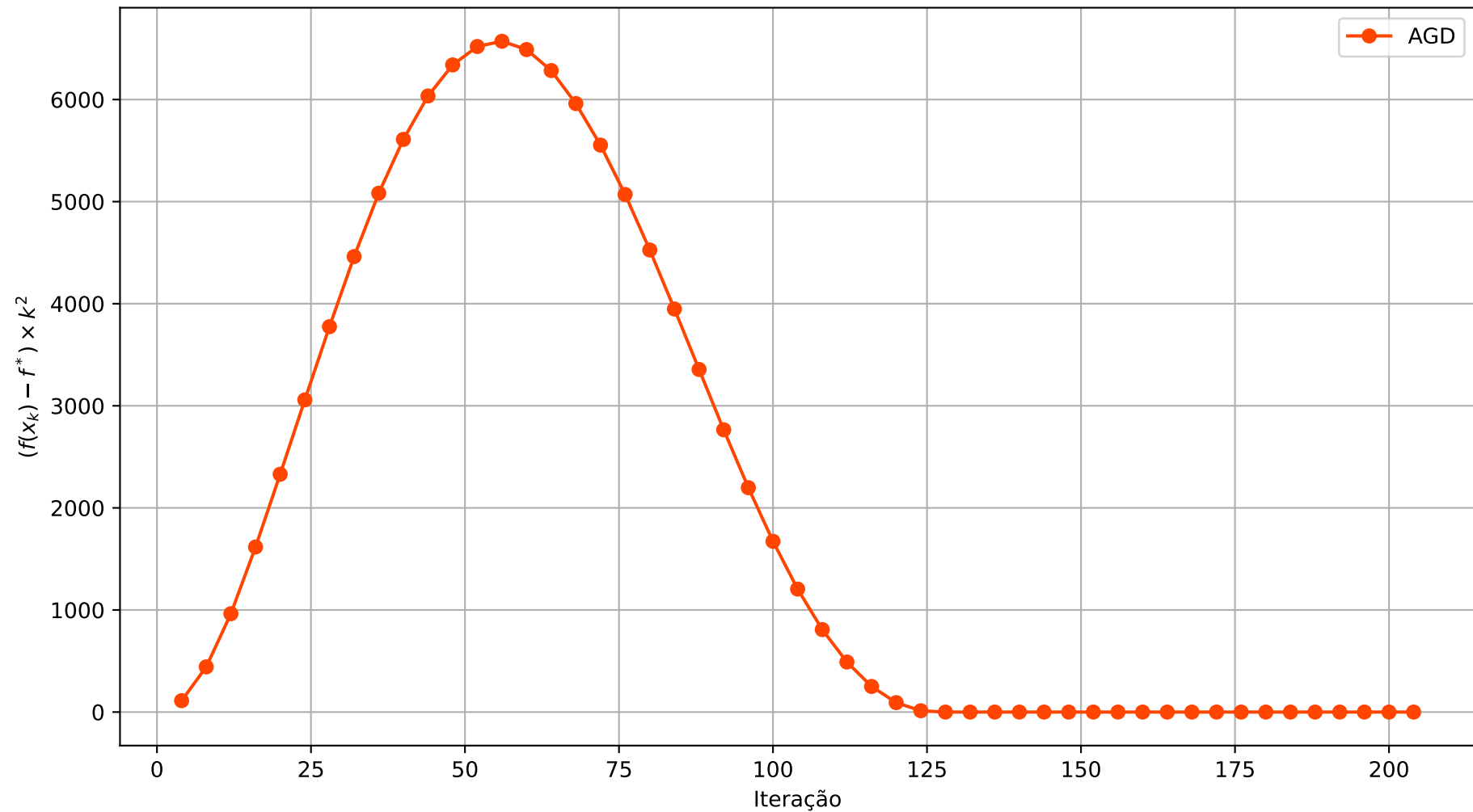
Verificação da taxa de convergência O(1/k^2) do AGD em dimensão 100
