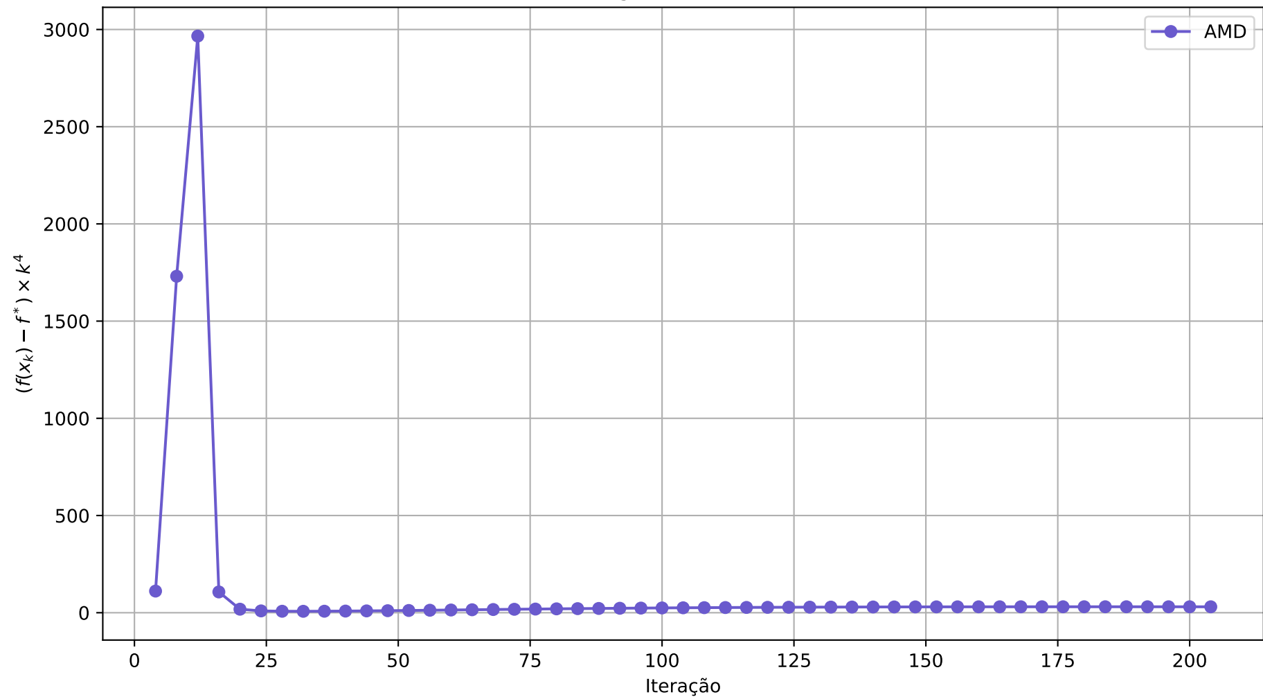
Verificação da taxa de convergência O(1/k^4) do AMD em dimensão 100
