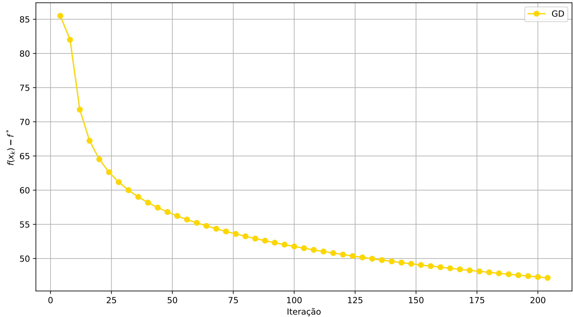
Verificação da taxa de convergência linear do GD em dimensão 100
