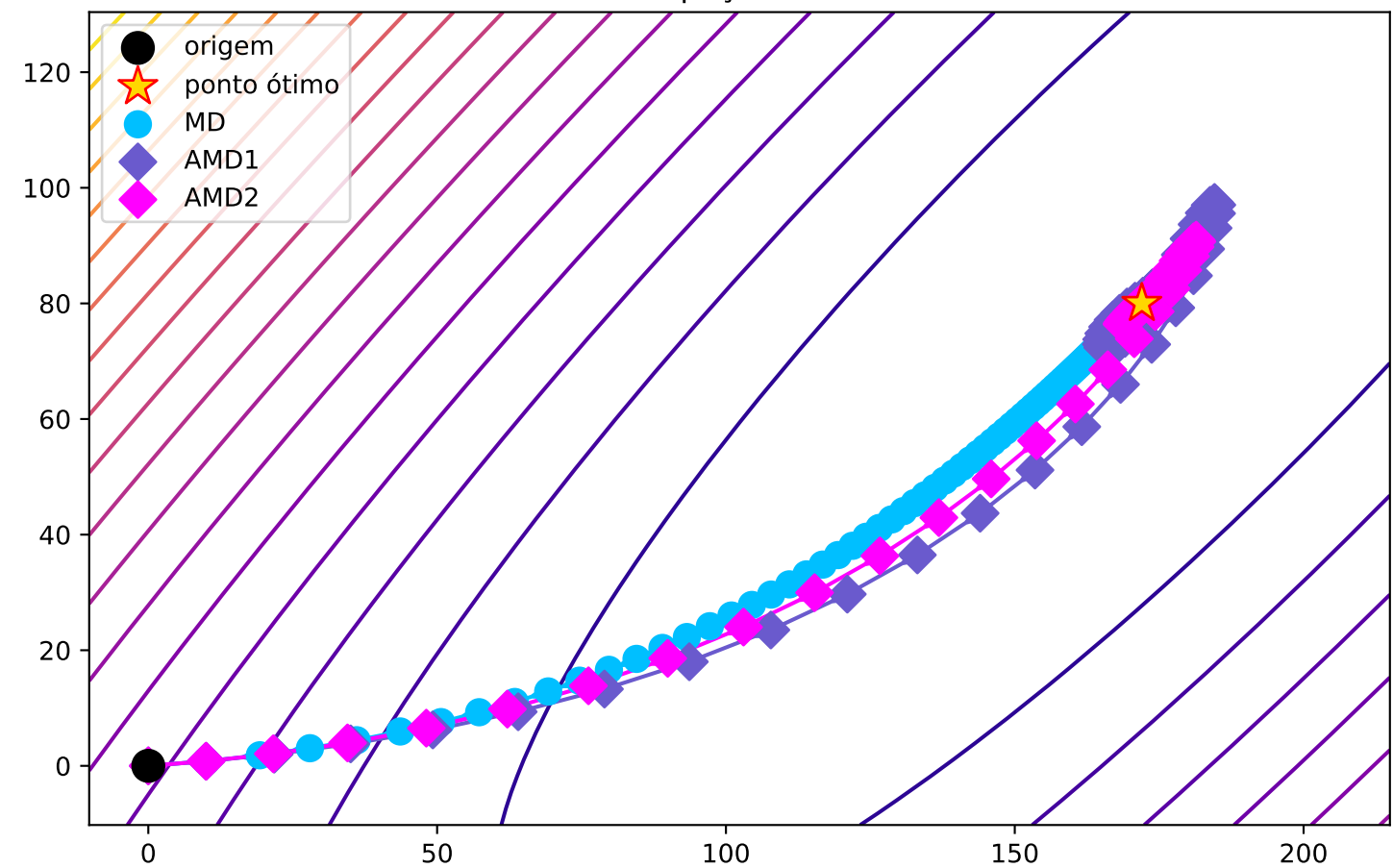
Espaço Dual
