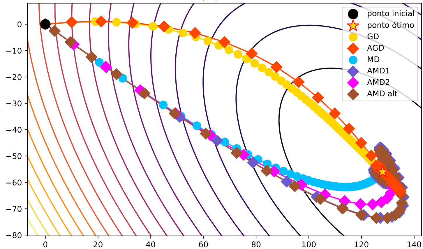
Espaço Primal
