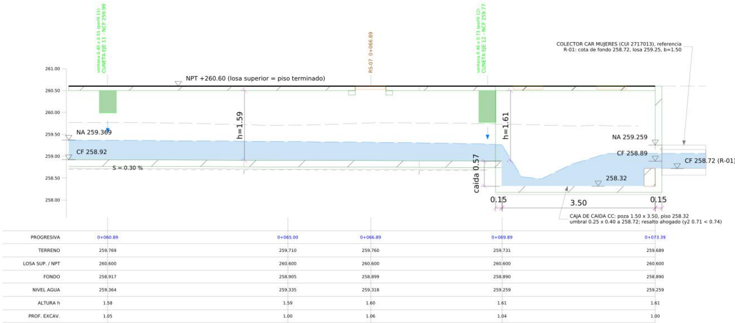
TRAMO 4: 0+060.00 A 0+073.39
