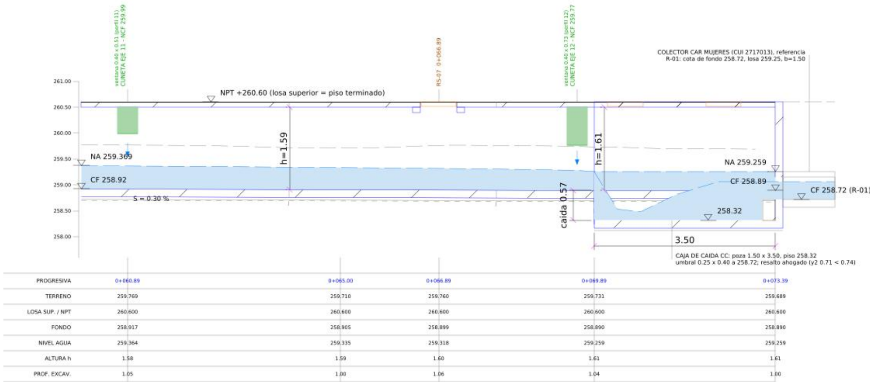
TRAMO 4: 0+060.00 A 0+073.39
