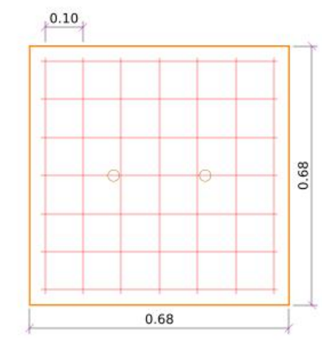
7 + 7 barras 3/8" @0.10, L=0.62; asas 3/8" liso
