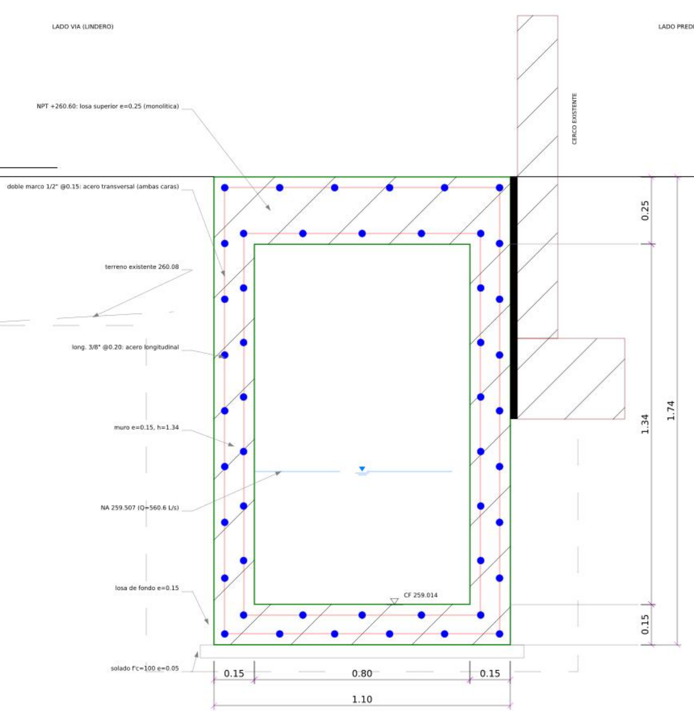
SECCION TIPICA C-C: CRUCE DE CAMIONES
