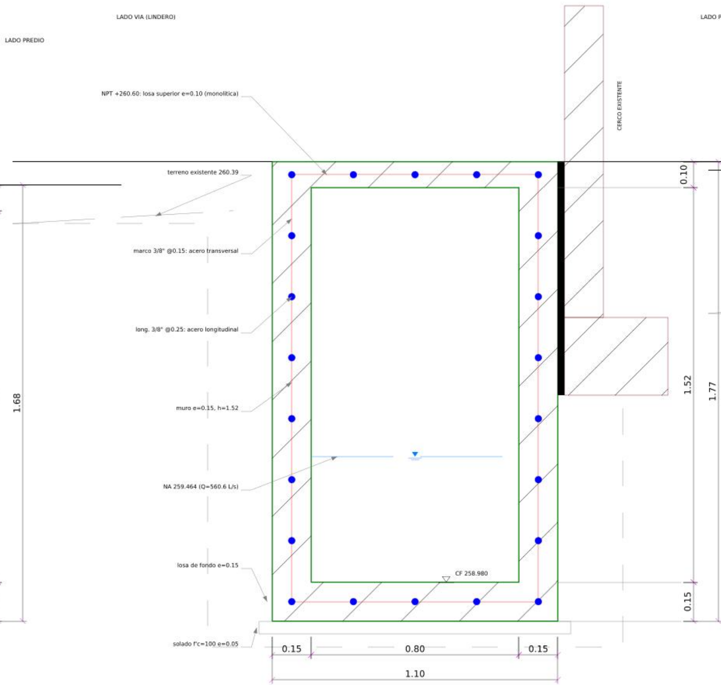
SECCION TIPICA B-B: CRUCE DE MOTOS
