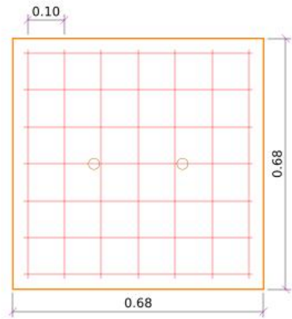
D. TAPA - ARMADO 7 + 7 barras 3/8" @0.10, L=0.62; asas 3/8" liso
