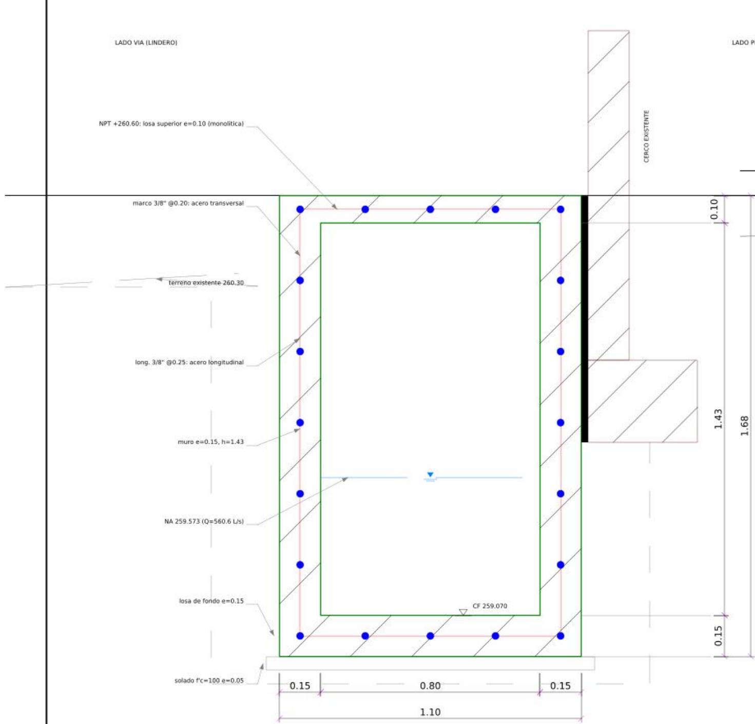
SECCION TIPICA A-A: TRAMO NORMAL
