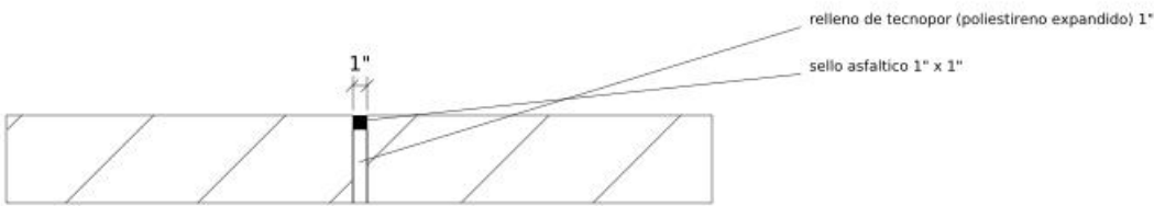
F. JUNTA DE DILATACION CADA 4.00 m
