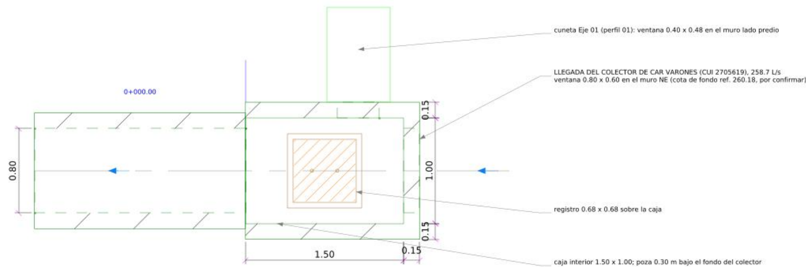
CL-1. CAJA DE LLEGADA - PLANTA
