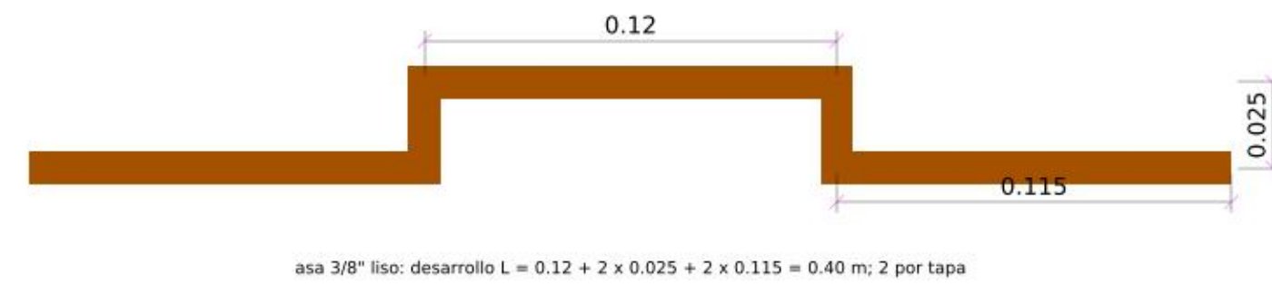
C. ASA DE IZAJE ESC. 1/2
