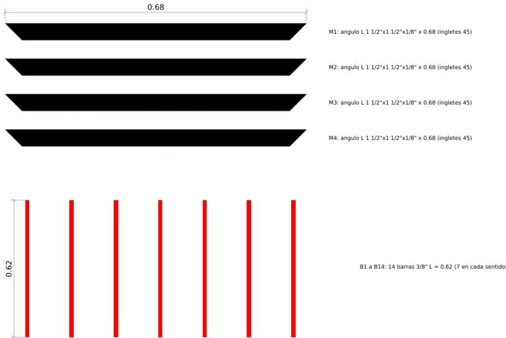
E. DESPIECE DEL MARCO Y DE LA PARRILLA ESC. 1/5 (barras acortadas en el dibujo)
