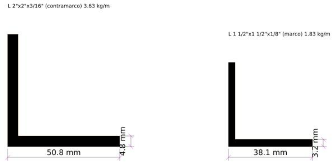
D. SECCIONES DE LOS ANGULOS ESC. 1/1
