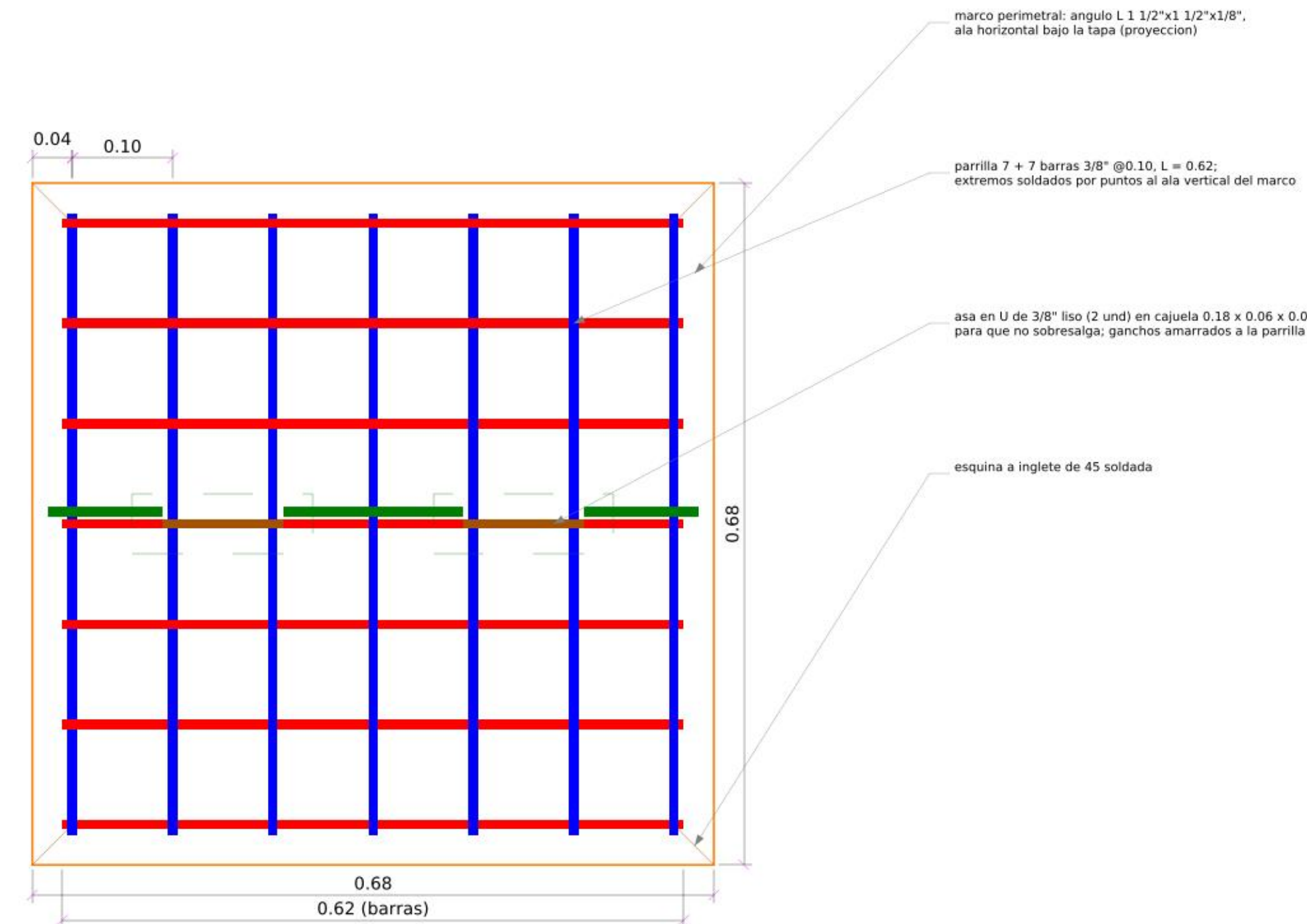
A. TAPA DE CONCRETO ARMADO - PLANTA (armado) ESC. 1/5 - 10 und (RS-01 a RS-07, CL y 2 en CC)
