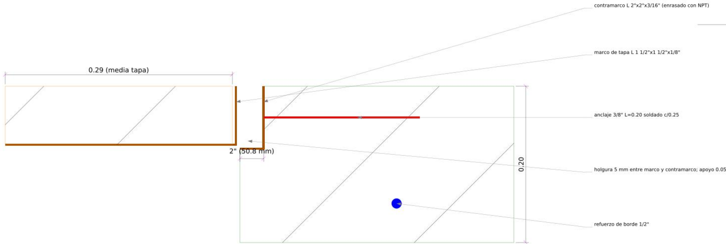
D. TAPA - CORTE
