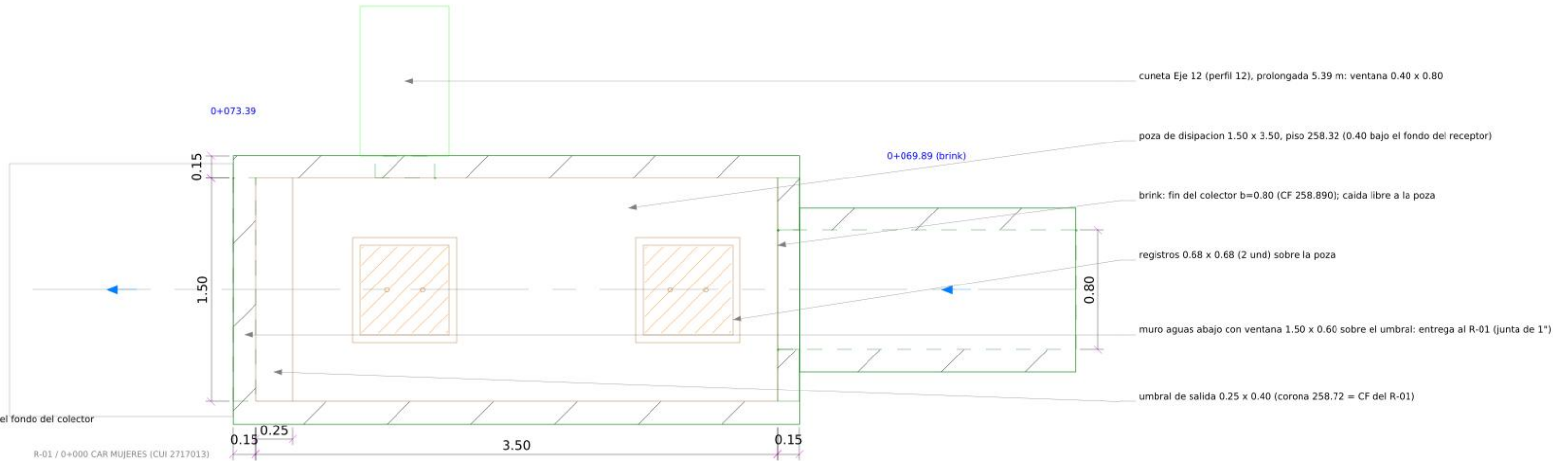
CC-1. CAJA DE CAIDA - PLANTA
