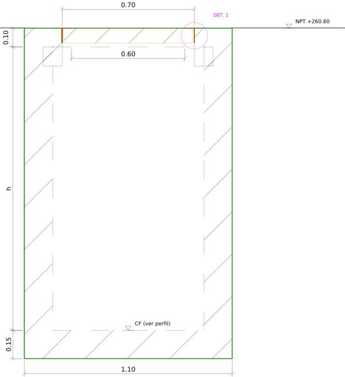
B. CORTE A-A POR EL REGISTRO
