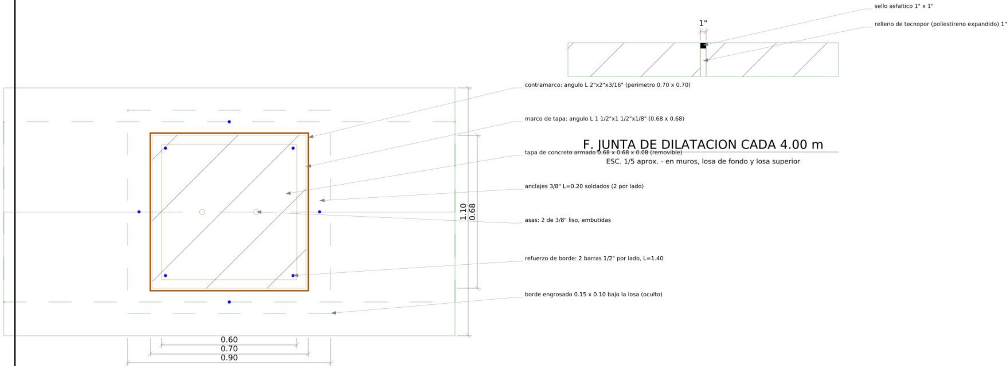
A. REGISTRO DE LIMPIEZA - PLANTA
