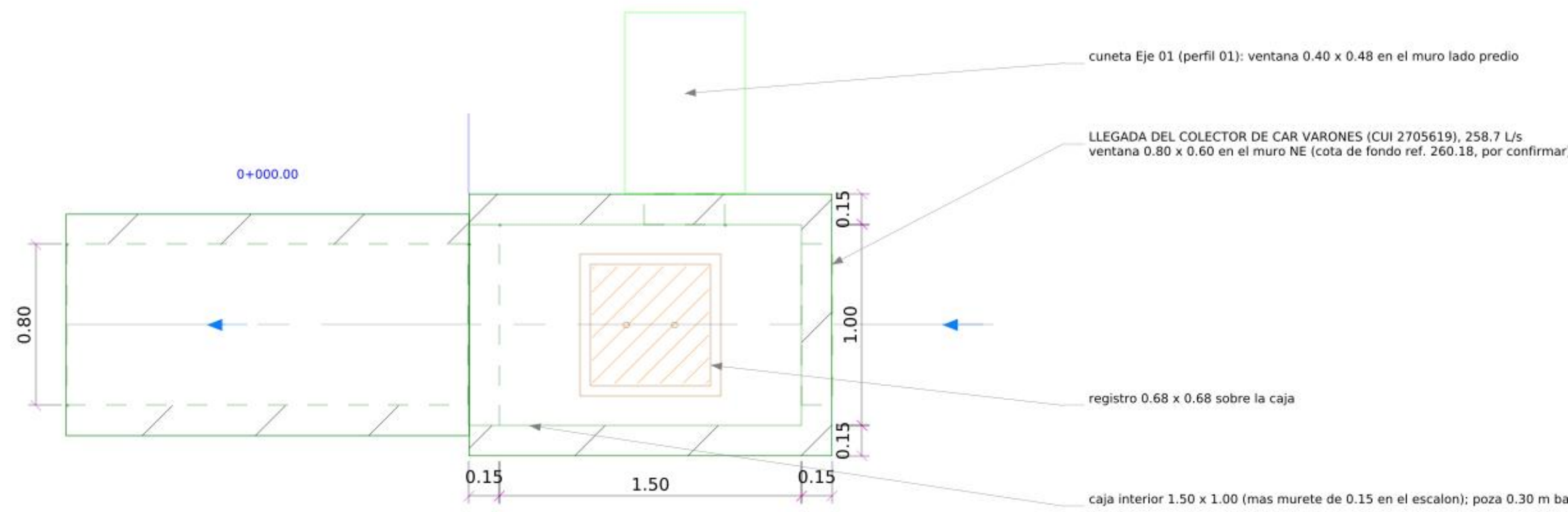
CL-1. CAJA DE LLEGADA - PLANTA
