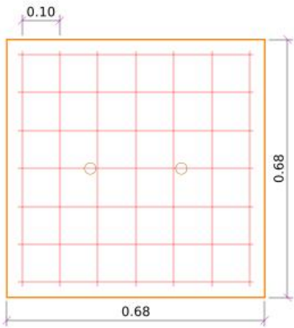
D. TAPA - ARMADO
