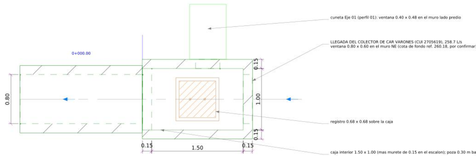
CL-1. CAJA DE LLEGADA - PLANTA
