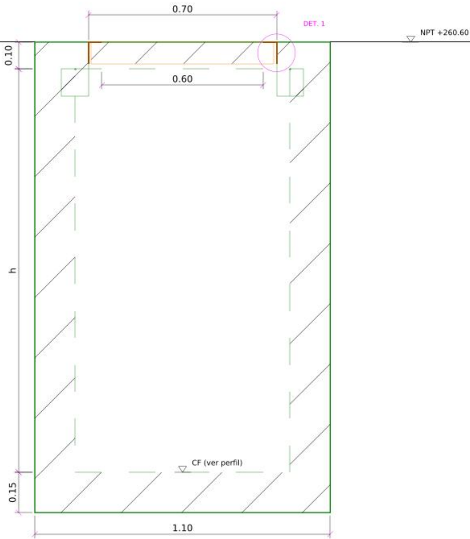
B. CORTE A-A POR EL REGISTRO
