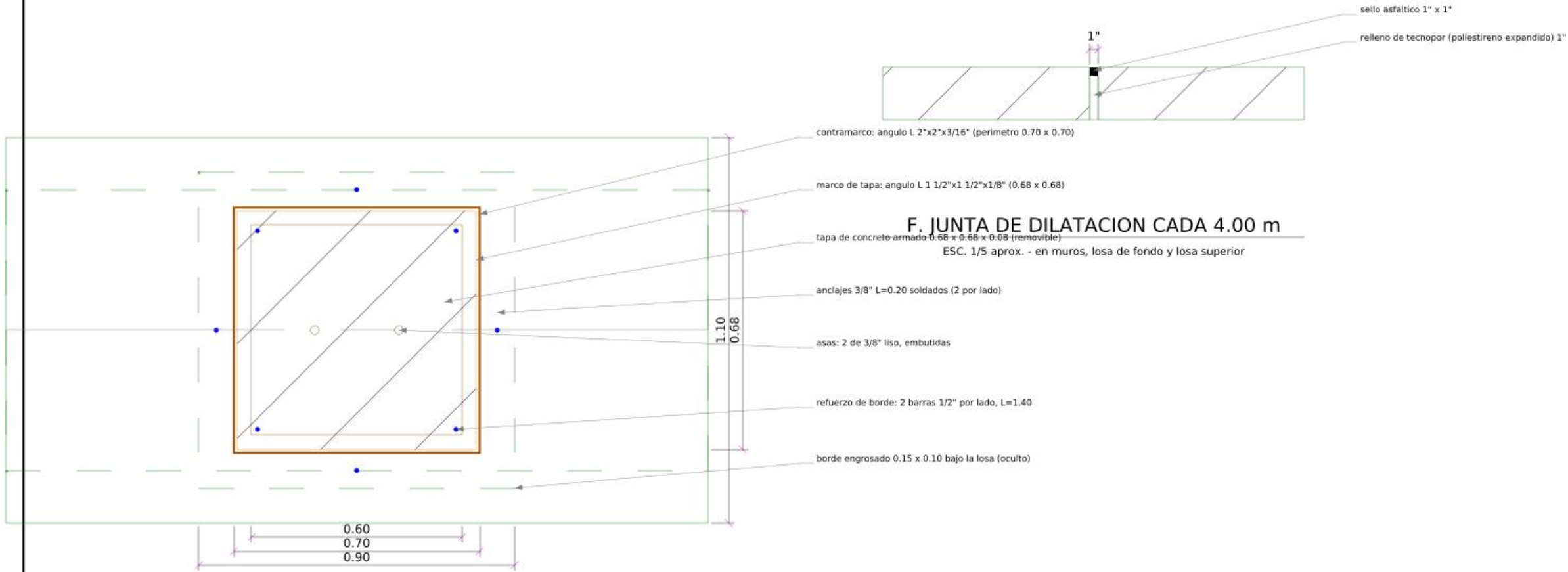
A. REGISTRO DE LIMPIEZA - PLANTA
