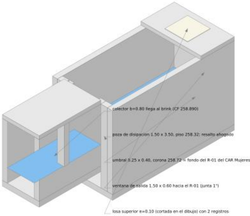
ISOMETRICO 4: CAJA DE CAIDA CON POZA
