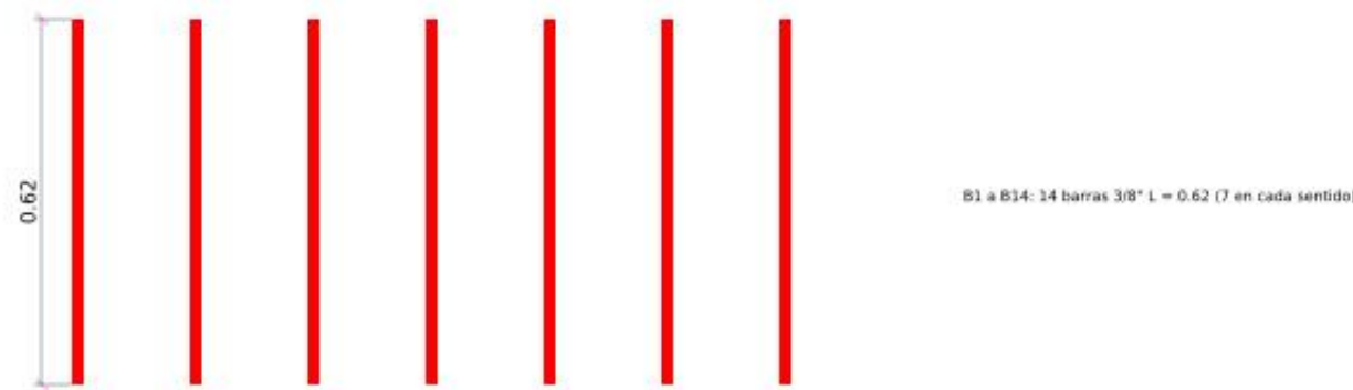
E. DESPIECE DEL MARCO Y DE LA PARRILLA ESC. 1/5 (barras acortadas en el dibujo)
