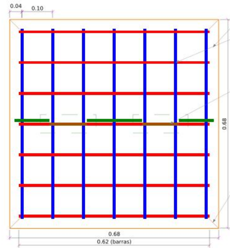
A. TAPA DE CONCRETO ARMADO - PLANTA (armado) ESC. 1/5 - 10 und (RS-01 a RS-07, CL y 2 en CC)
