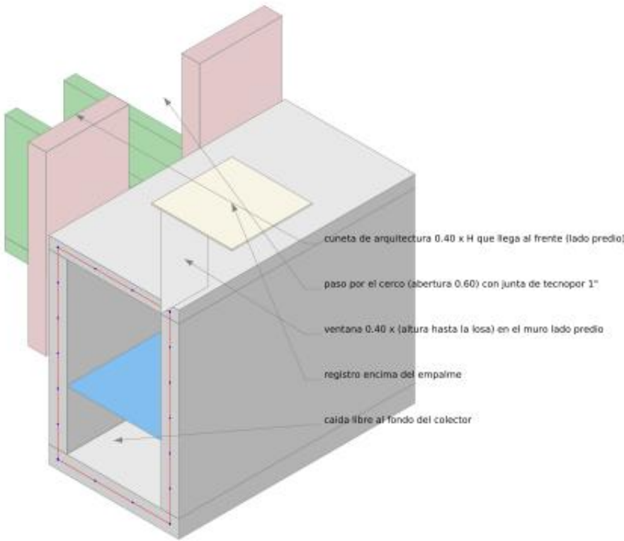
ISOMETRICO 3: EMPALME DE CUNETA
