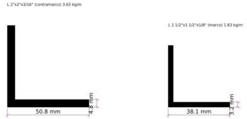
D. SECCIONES DE LOS ANGULOS ESC. 1/1
