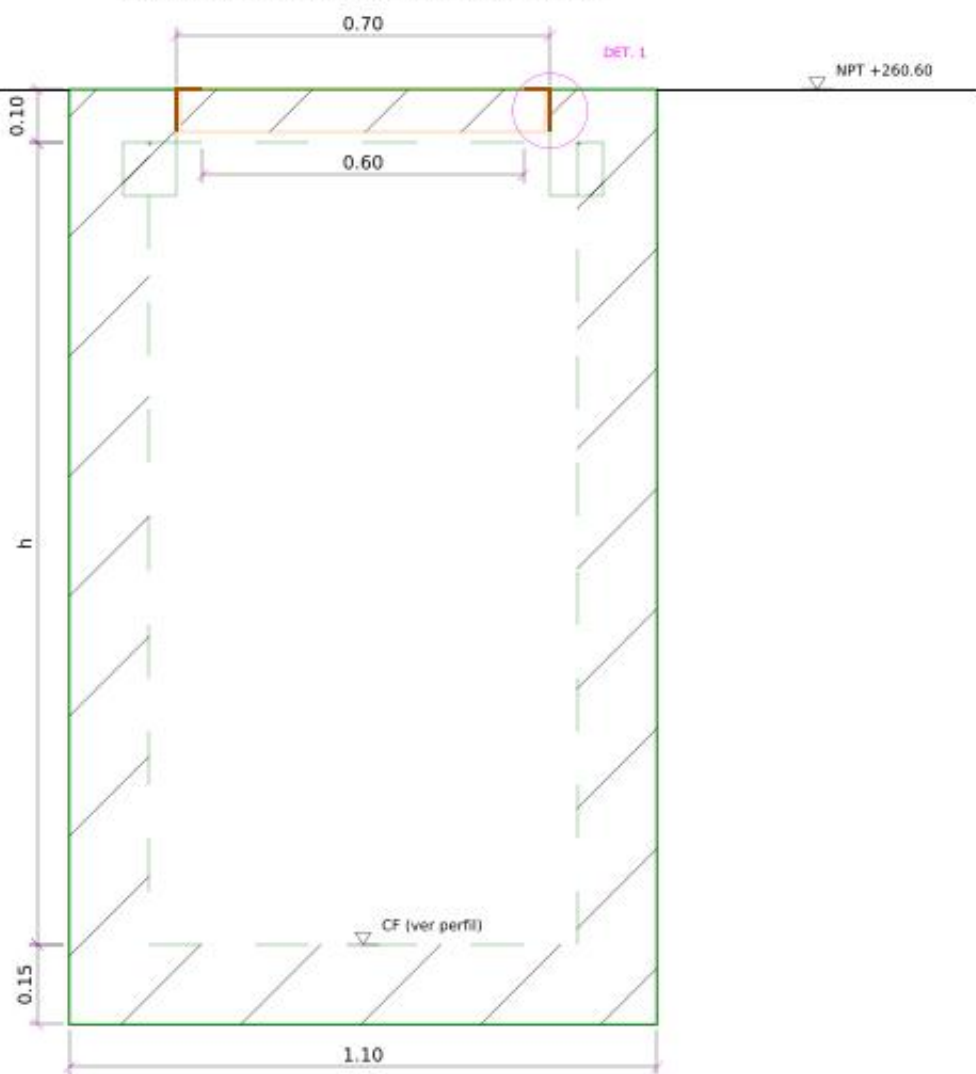
B. CORTE A-A POR EL REGISTRO ESC. 1/10
