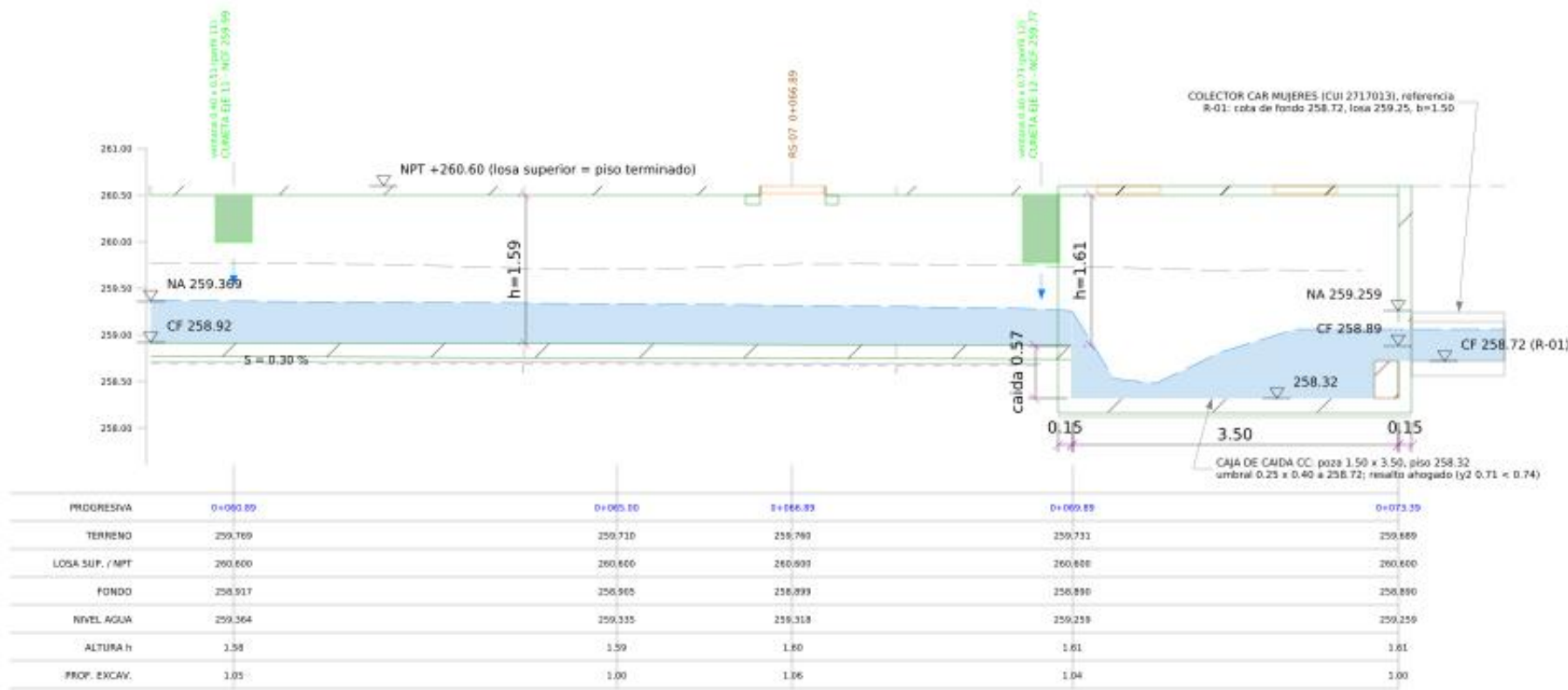
TRAMO 4: 0+060.00 A 0+073.39
