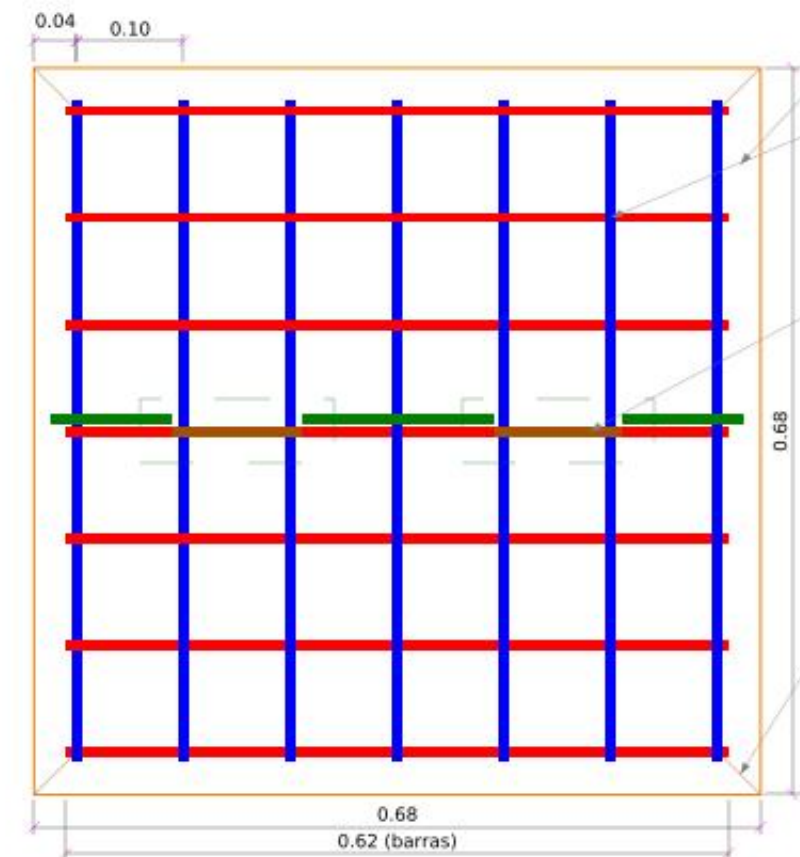
A. TAPA DE CONCRETO ARMADO - PLANTA (armado) ESC. 1/5 - 11 und (RV-01 a RV-11)
