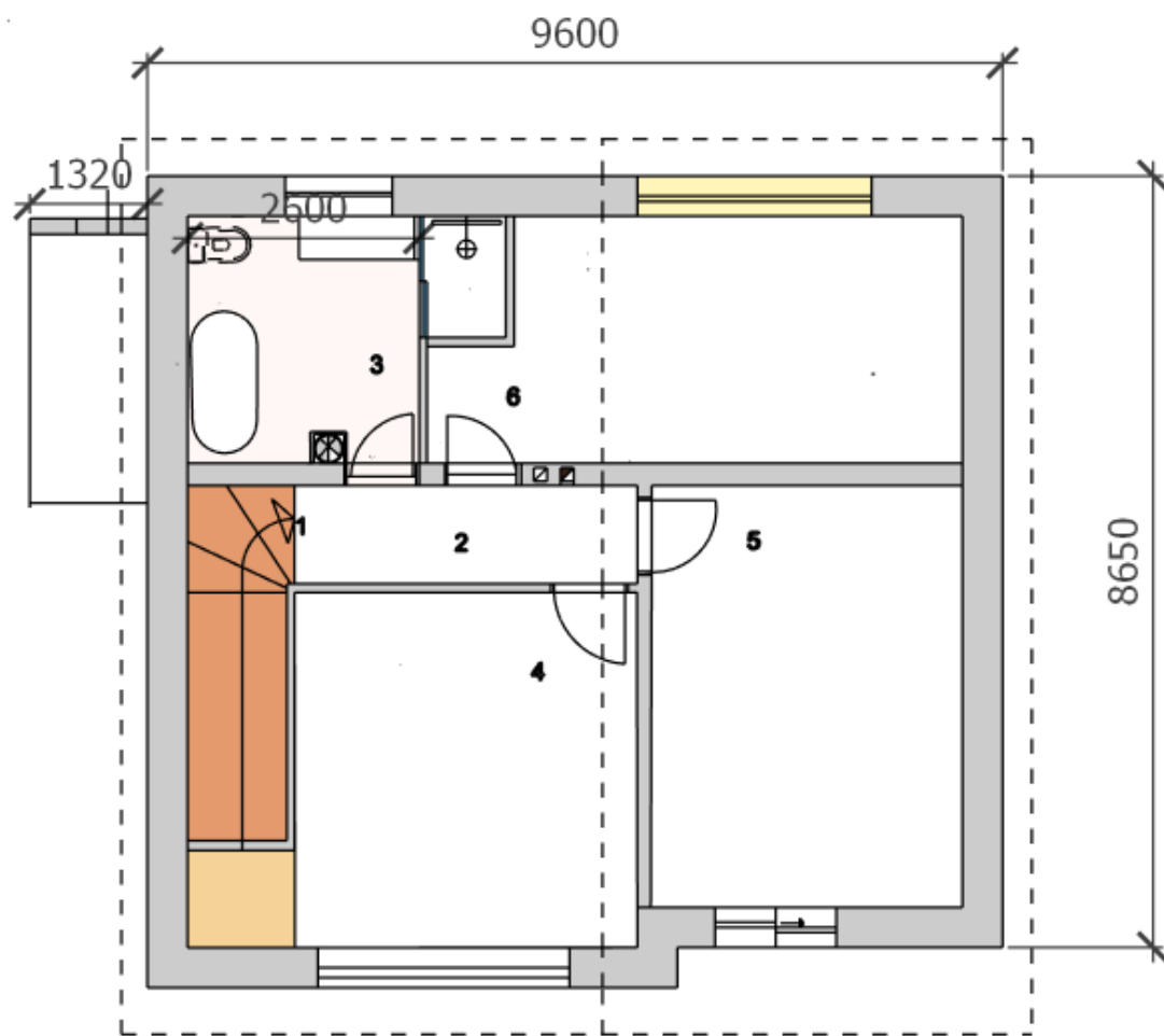
PODLAŽÍ 2NP – BEZE ZMEN
